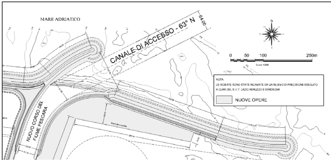
Figura 2.4 – Foce fiume Pescara: planimetria di progetto con l'indicazione del canale di accesso
