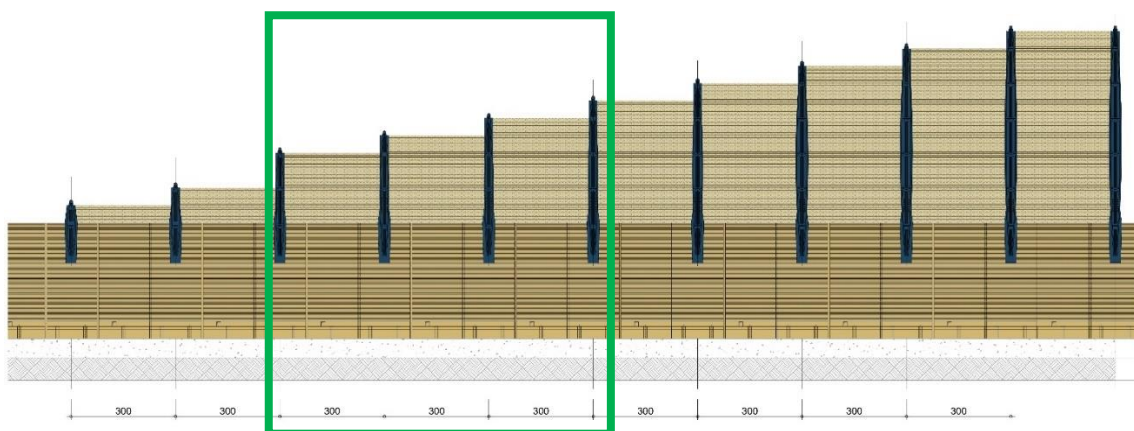
Figura 2-34 - Sezione tipologica delle barriere antirumore (in verde i moduli previsti per il presente progetto)
