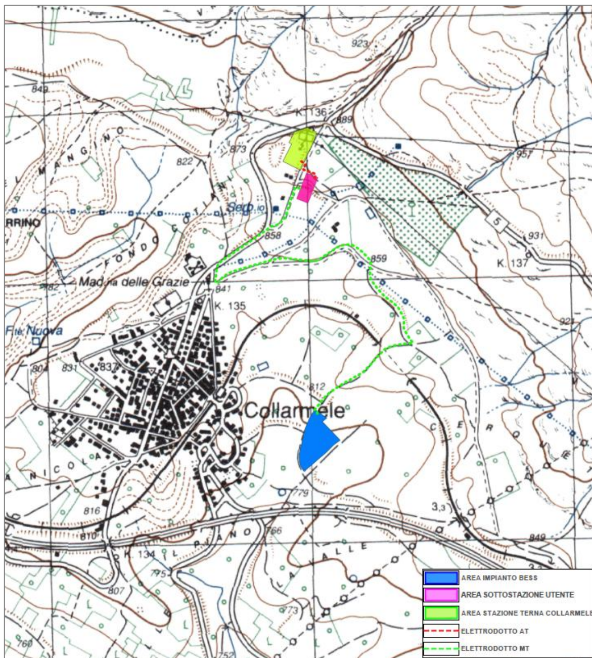
Figura 6 – Area impianto e cavidotto su IGM 1:10.000
