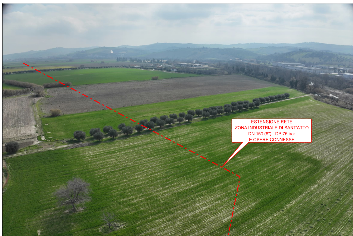
FOTO 22: Percorrenza nei campi
