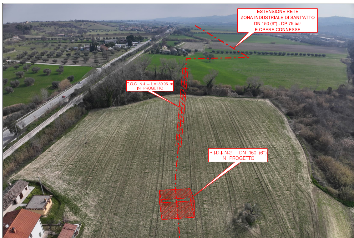
FOTO 21: Percorrenza nei campi e attraversamento Torrente Ceca mediante Trivellazione Orizzontale Controllata (T.O.C. N.4 L=180m)
