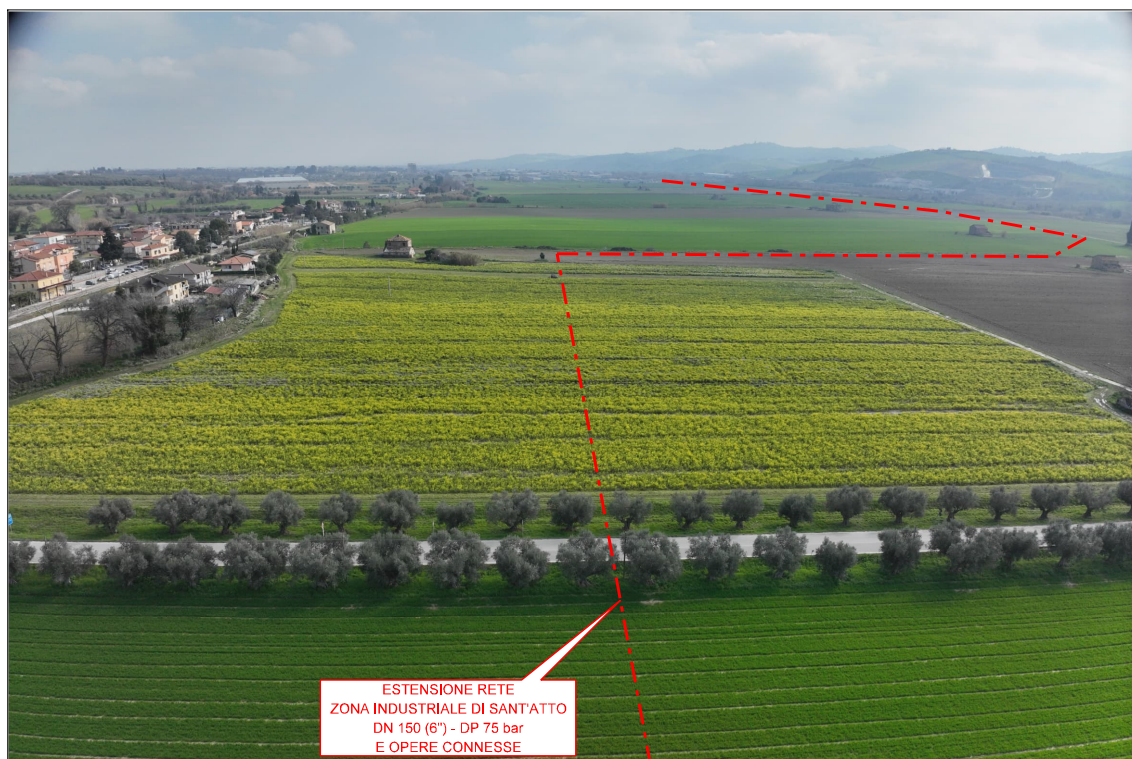
FOTO 24: Percorrenza nei campi e attraversamento S.S. N.553
