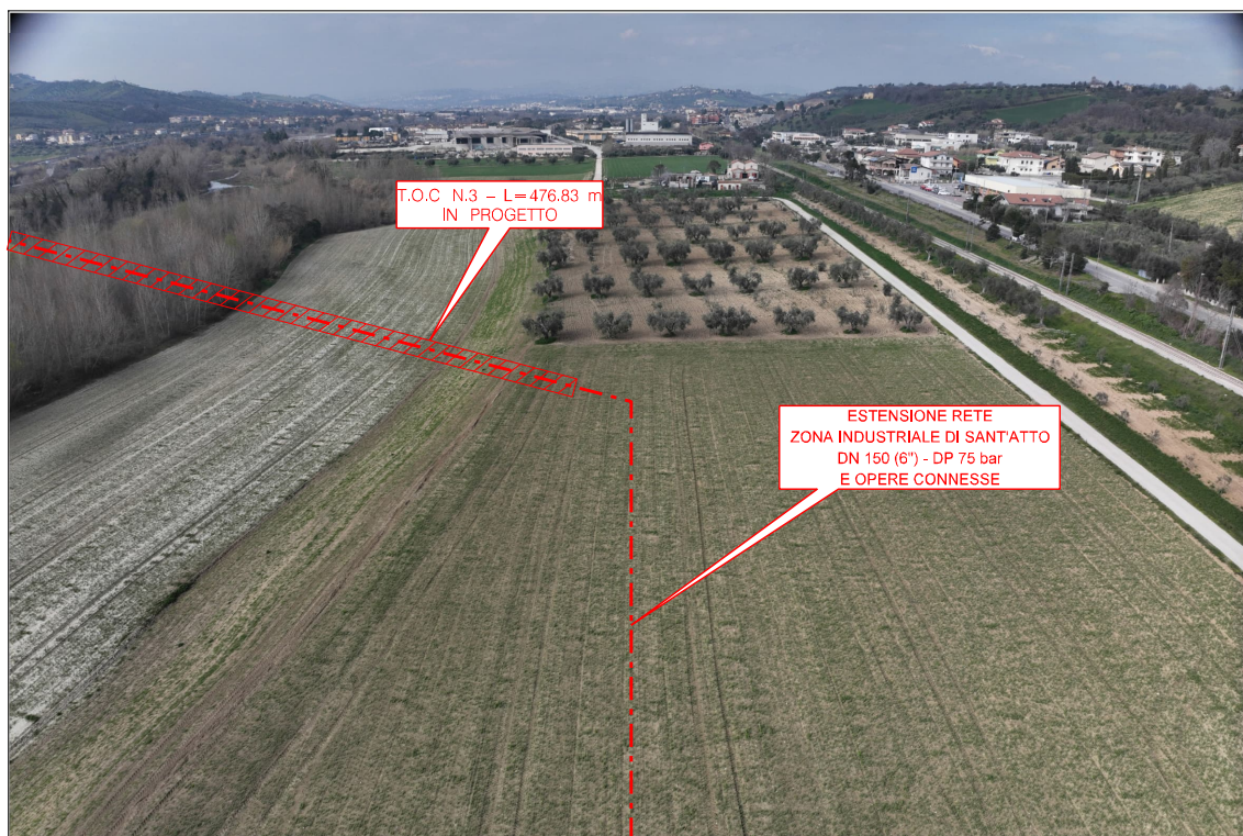
FOTO 19: Percorrenza nei campi e secondo attraversamento Fiume Tordino mediante Trivellazione Orizzontale Controllata (T.O.C. N.3 L=480m)
