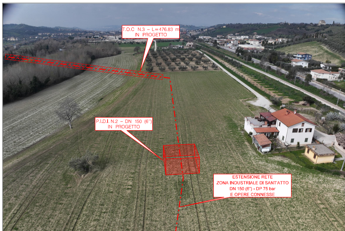
FOTO 20: Vista panoramica secondo attraversamento Fiume Tordino e ubicazione Impianto P.I.D.I. N.2 DN 150 (6") x DN 100 (4)
