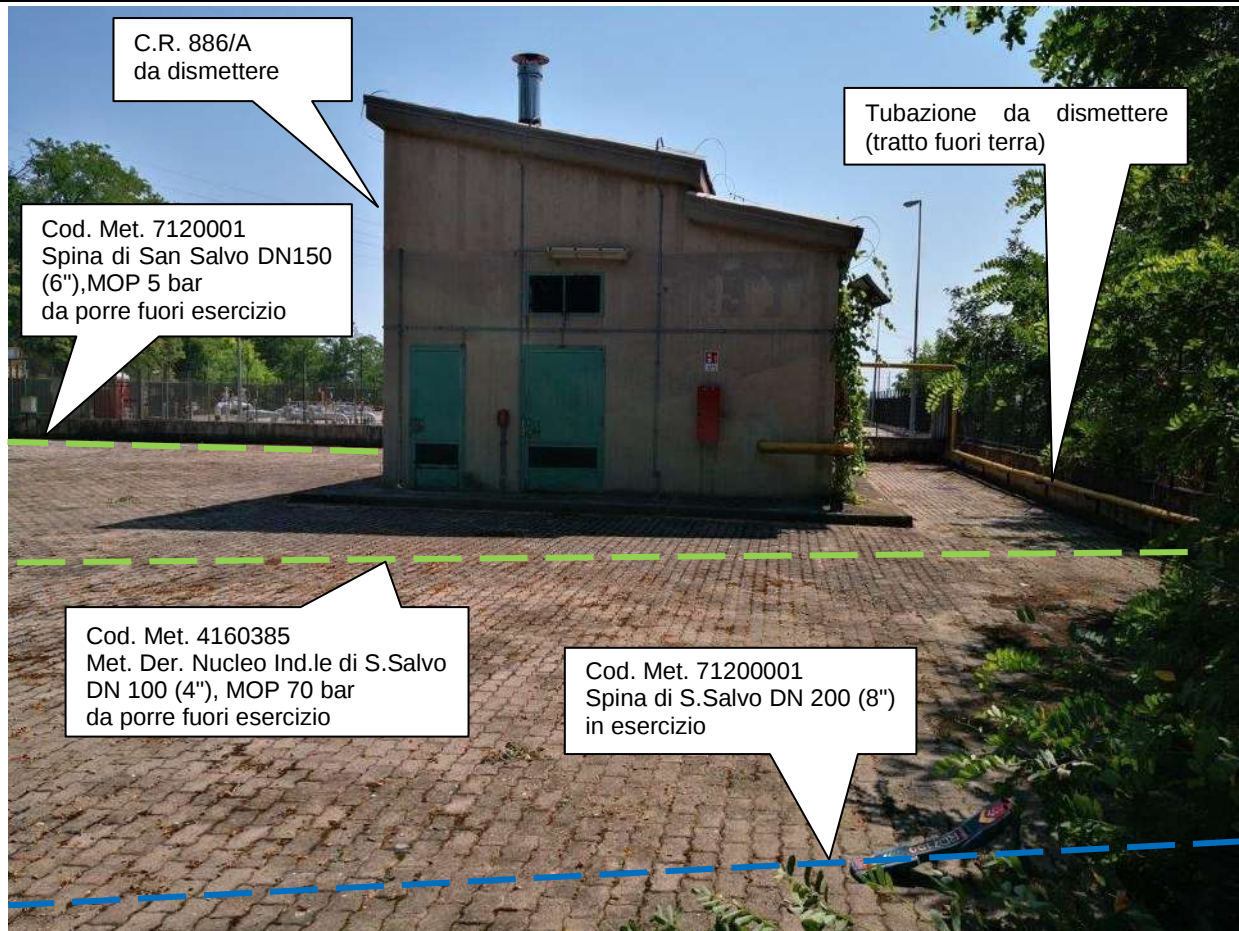
Foto 16- dismissione cabina di riduzione 886/A
