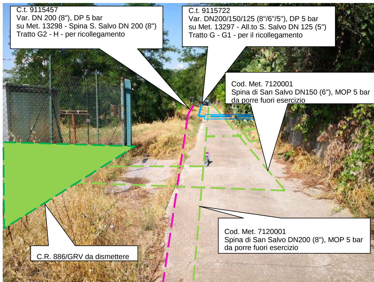
Foto 9 – dismissione cabina 886-GRV e stacchi ai metanodotti oggetto di variante
