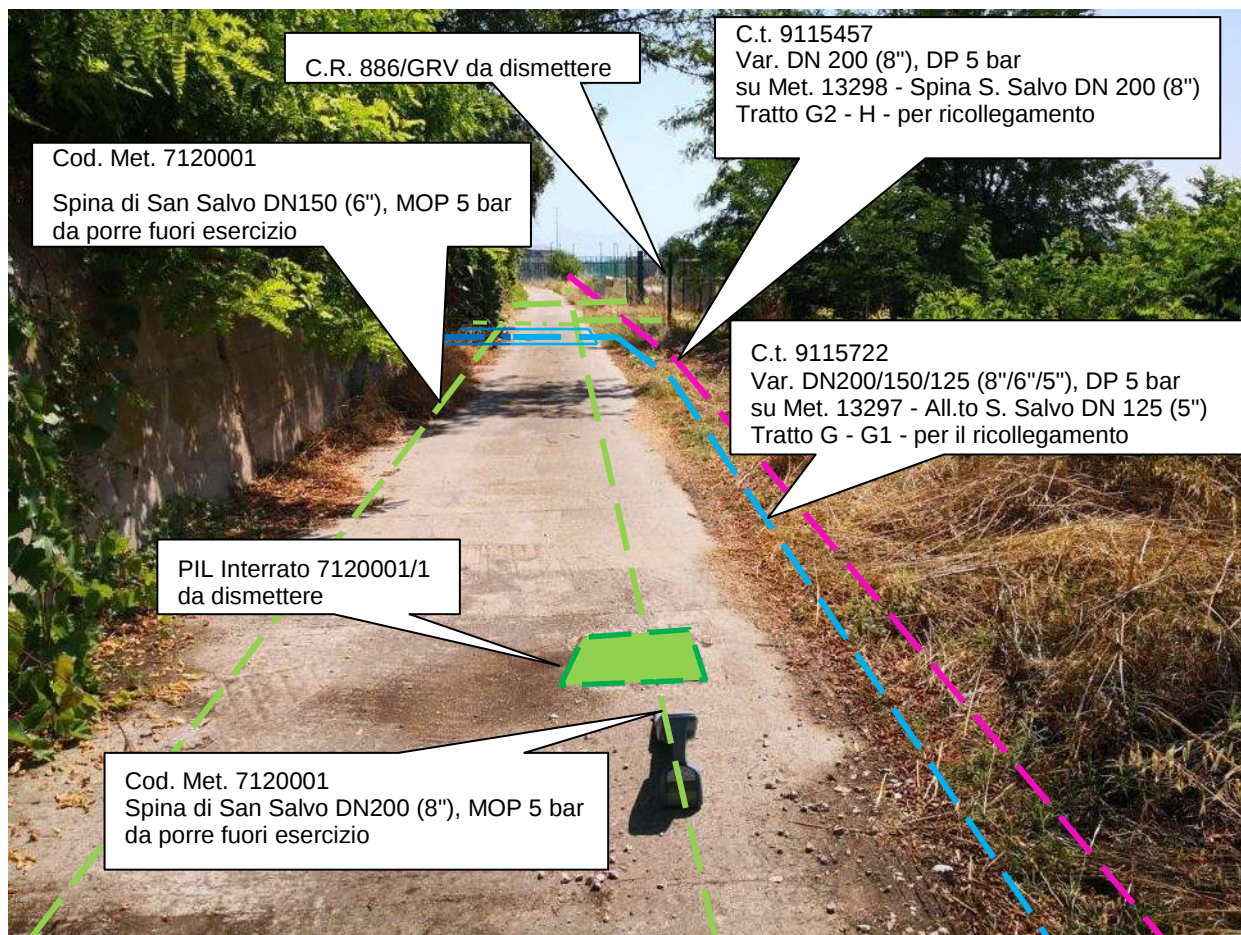
Foto 10 – dismissione valvola in pozzetto N-7120001/1 – tratto di variante DN 200 e DN 150 in parallelismo
