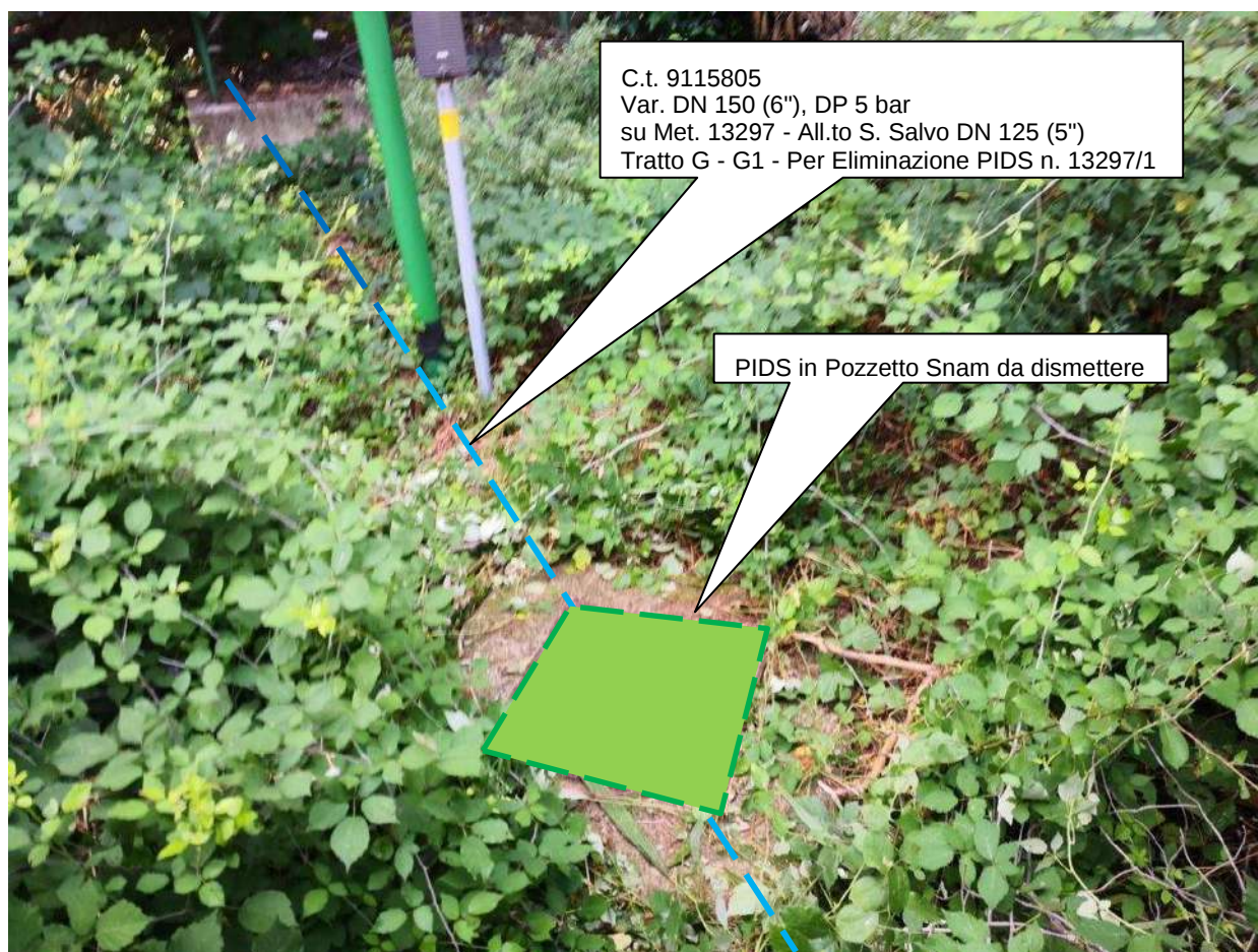
Foto 6 – dismissione valvola in pozzetto n.13297/1
