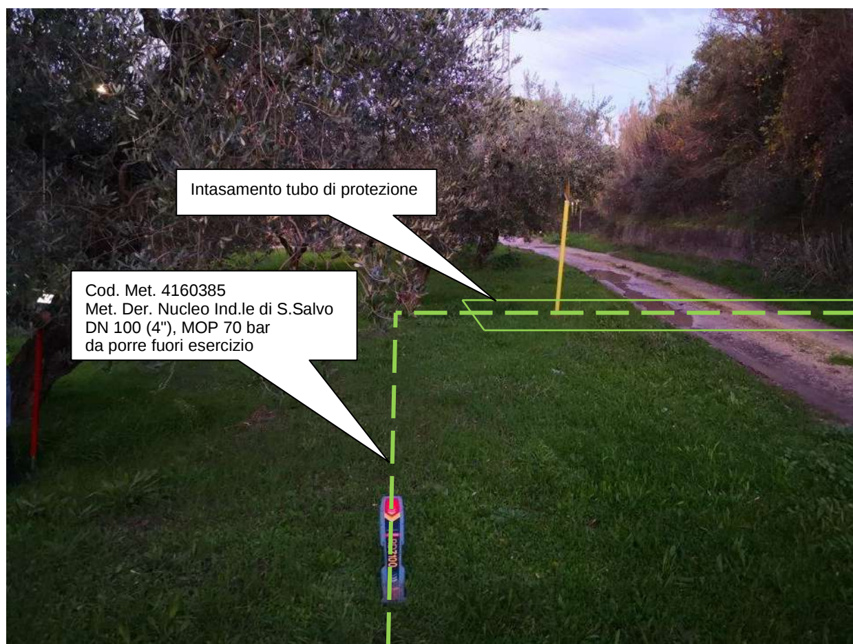
Foto 4 – dismissione metanodotto 4160385 e intasamento tubo di protezione
