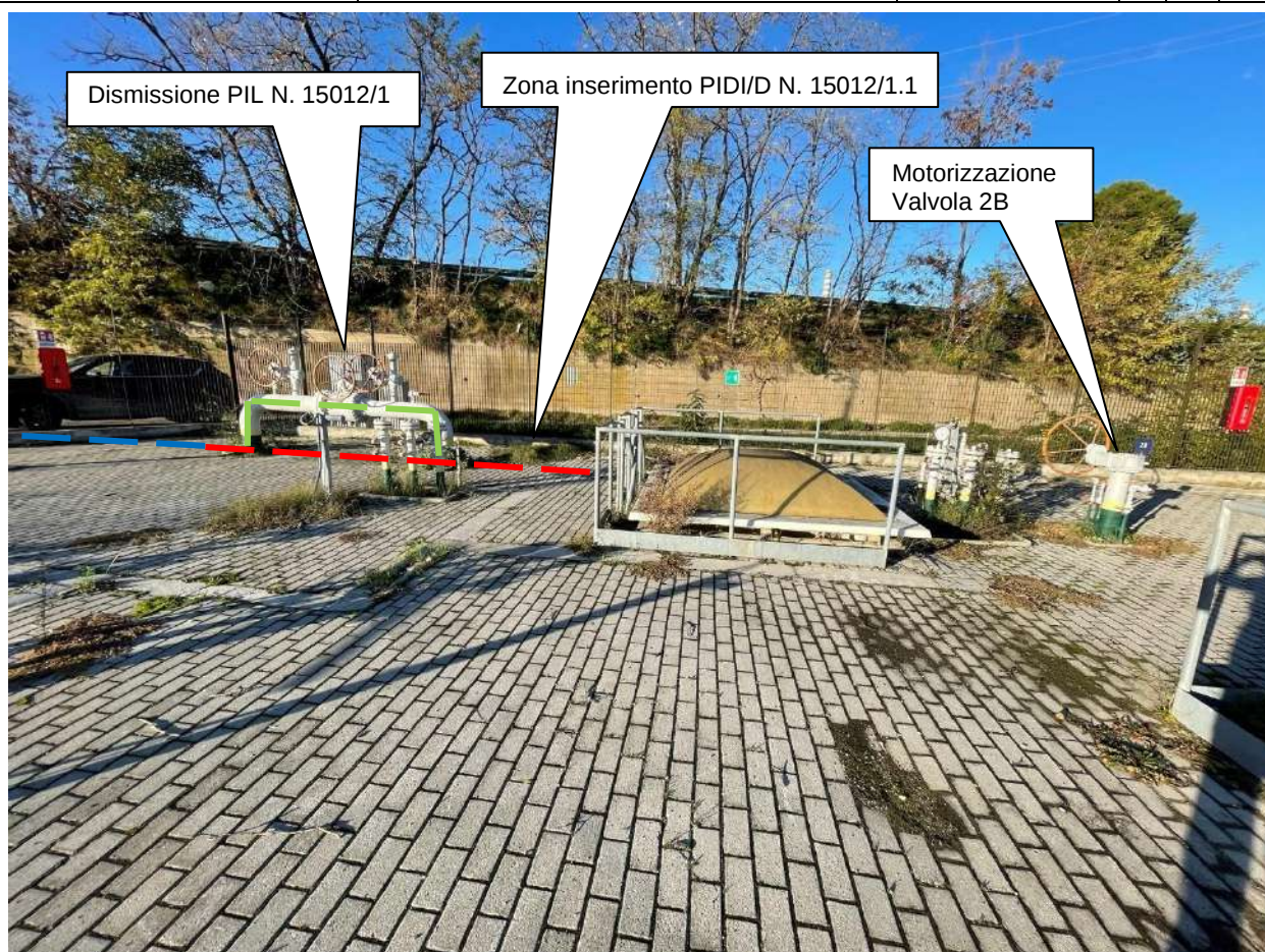
Foto 13 – motorizzazione valvola 2B – dismissione PIL N. 15012/1- inserimento PIDI/D N. 15012/1.1
