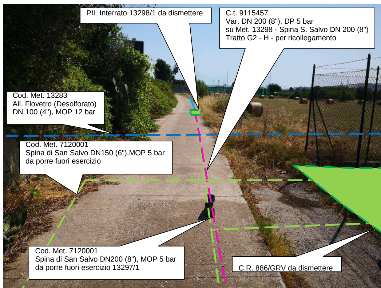
Foto 8 – dismissione cabina 886-GRV- valvola in pozzetto n.13298/1
