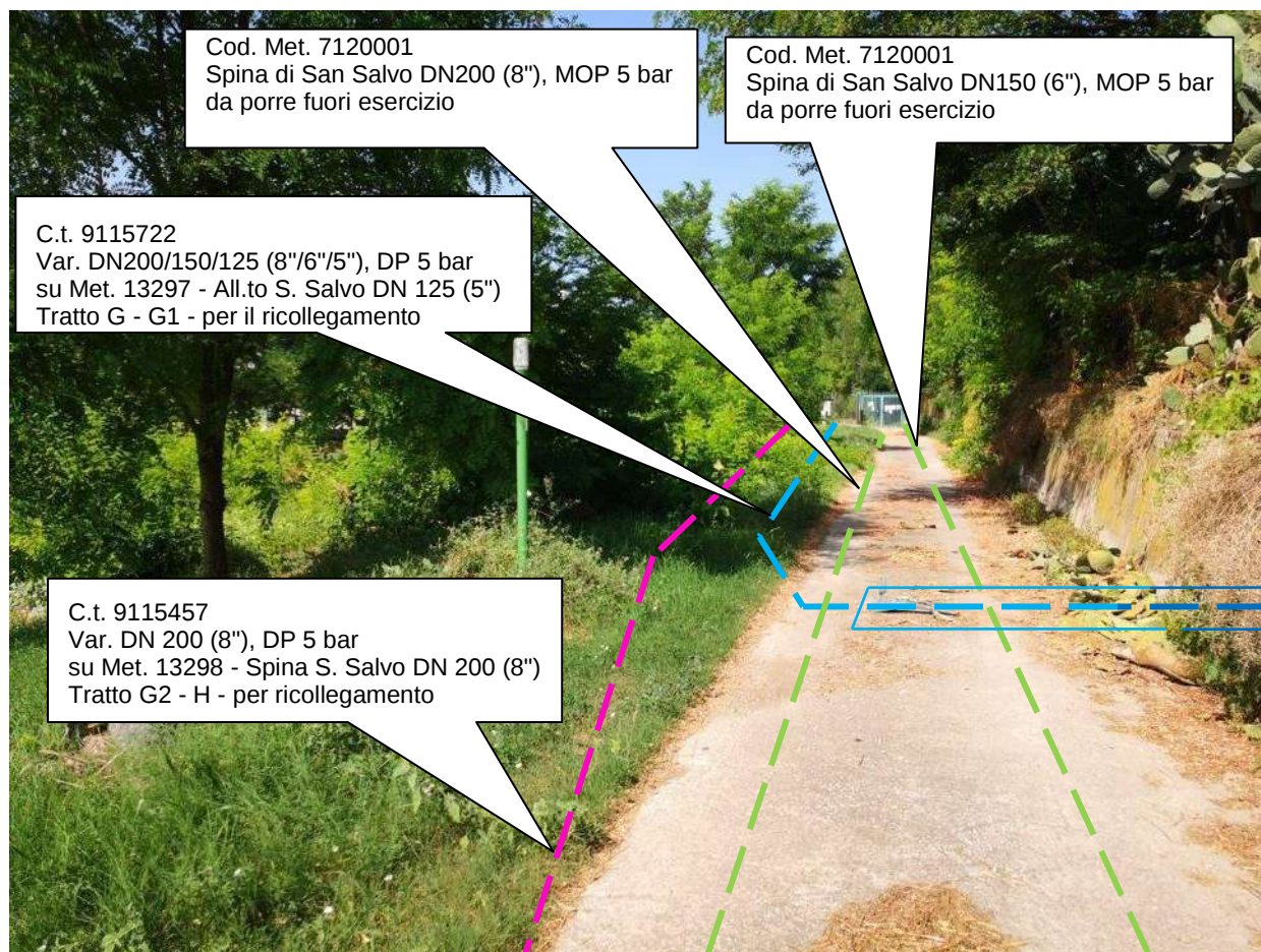
Foto 5 – Variante ricollegamento metanodotto N. 13297 – Fine tratto di parallelismo col metanodotto N.13298
