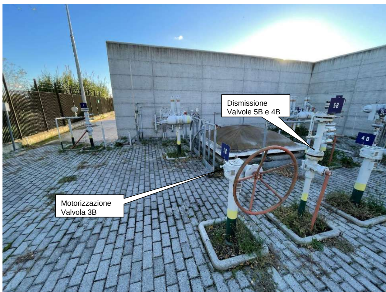
Foto 12 – motorizzazione Valvola 3B – dismissione Valvole
