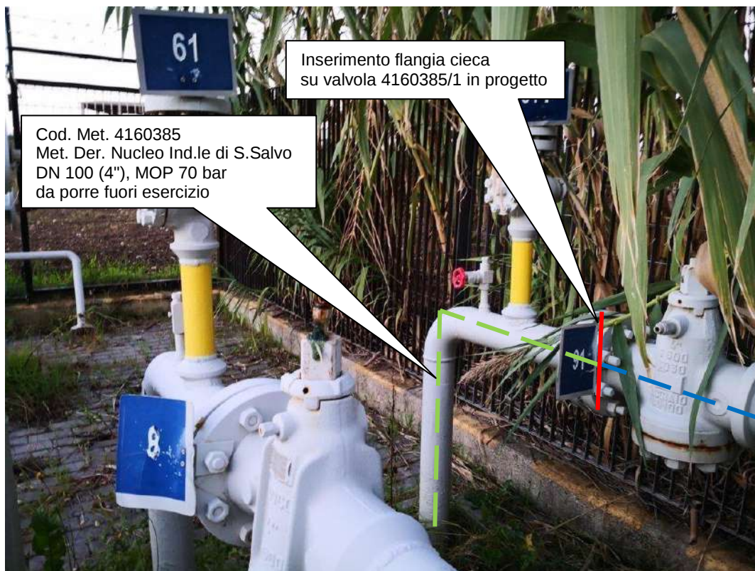
Foto 1 – Inserimento flangia su valvola n 91 impianto N. 4160385/1
