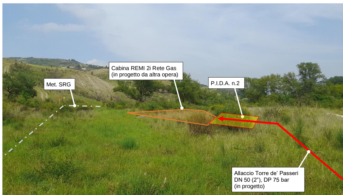
Foto n. 4 – Punto terminale, PIDA n.2 in progetto e cabina REMI 2iRG in progetto da altra opera
