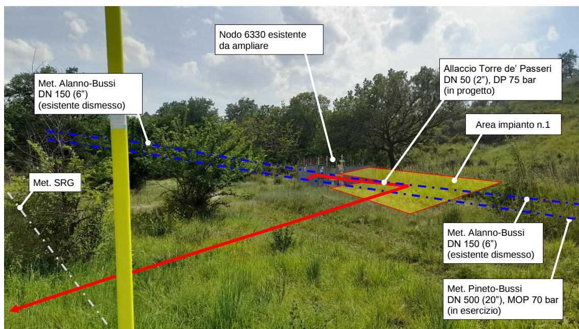
Foto n. 1 - Area impianto n.1 (Nodo 6330 da ampliare)
