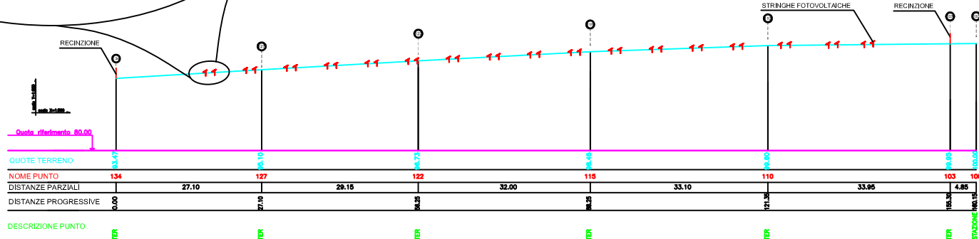
Sezione Longitudinale "A"
