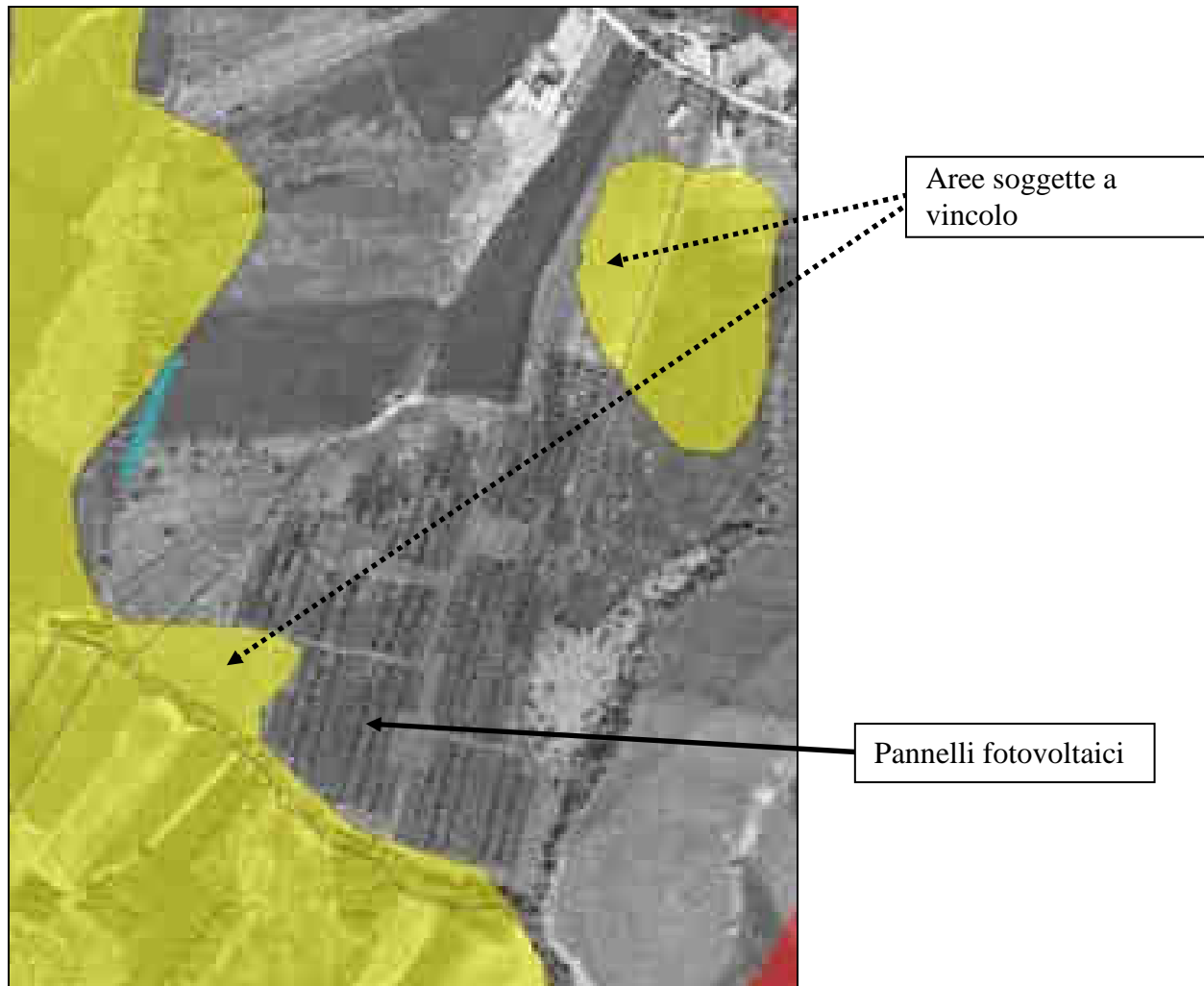
Figura 8 – Localizzazione dell’impianto fotovoltaico rispetto alle aree sottoposte a vincolo Fonte: Nostra elaborazione su dati del Piano Stralcio di Bacino per l’Assetto Idrogeologico Carta del vincolo idrogeologico
