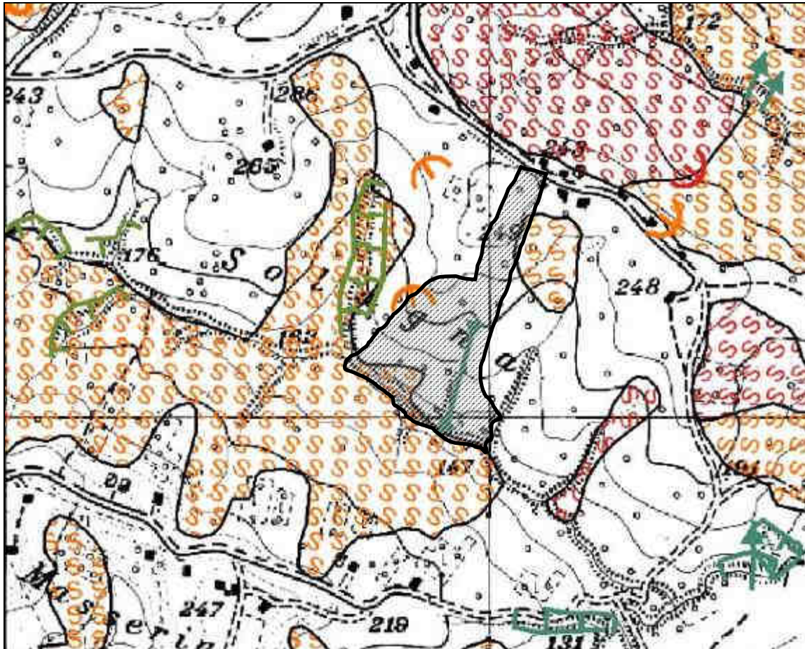
Figura 7 - Piano stralcio di bacino per l'assetto idrogeologico - Carta inventario dei fenomeni franosi ed erosivi
