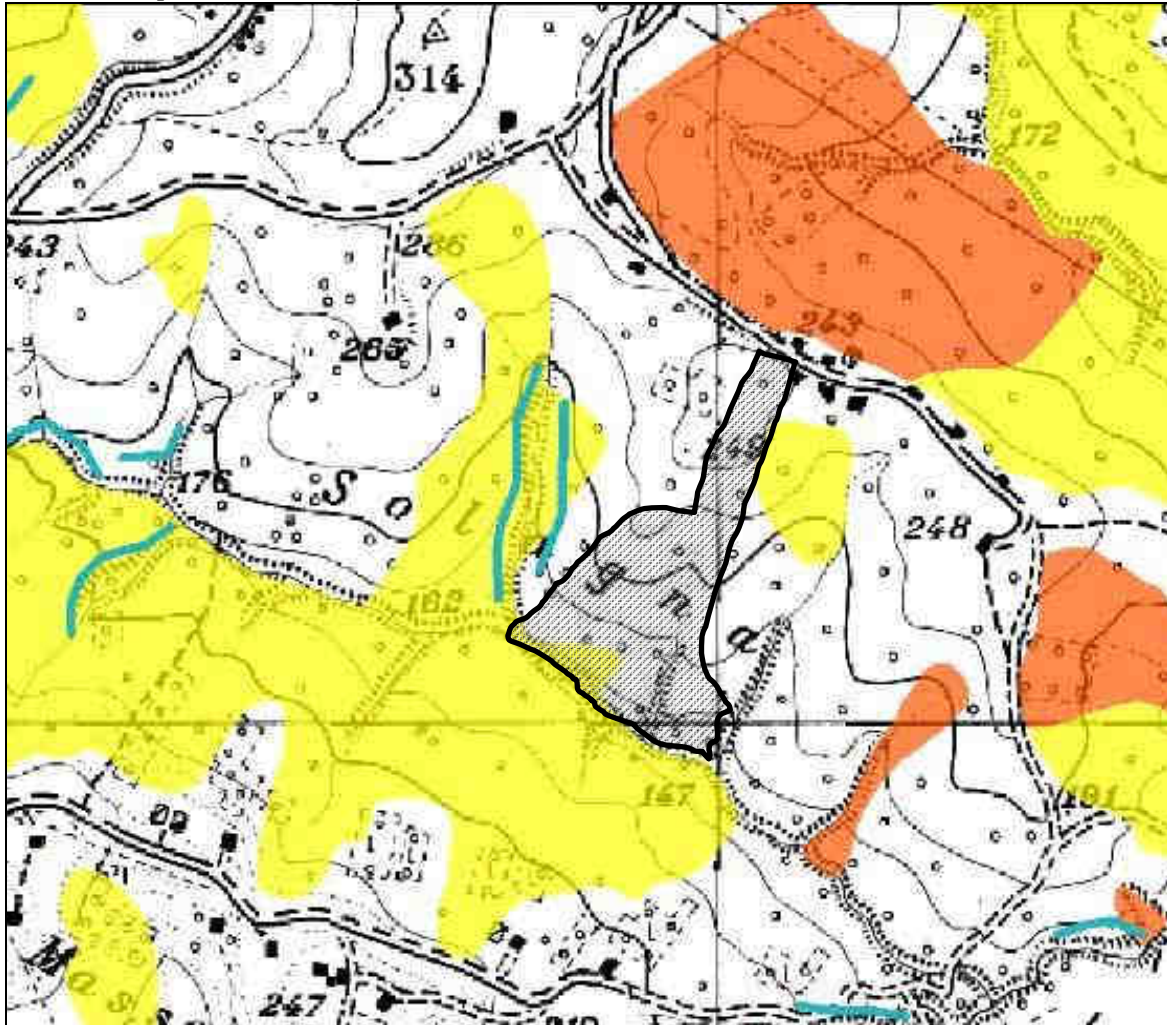
Figura 10 - Piano stralcio di bacino per l'assetto idrogeologico - Carta della pericolosità da frana
