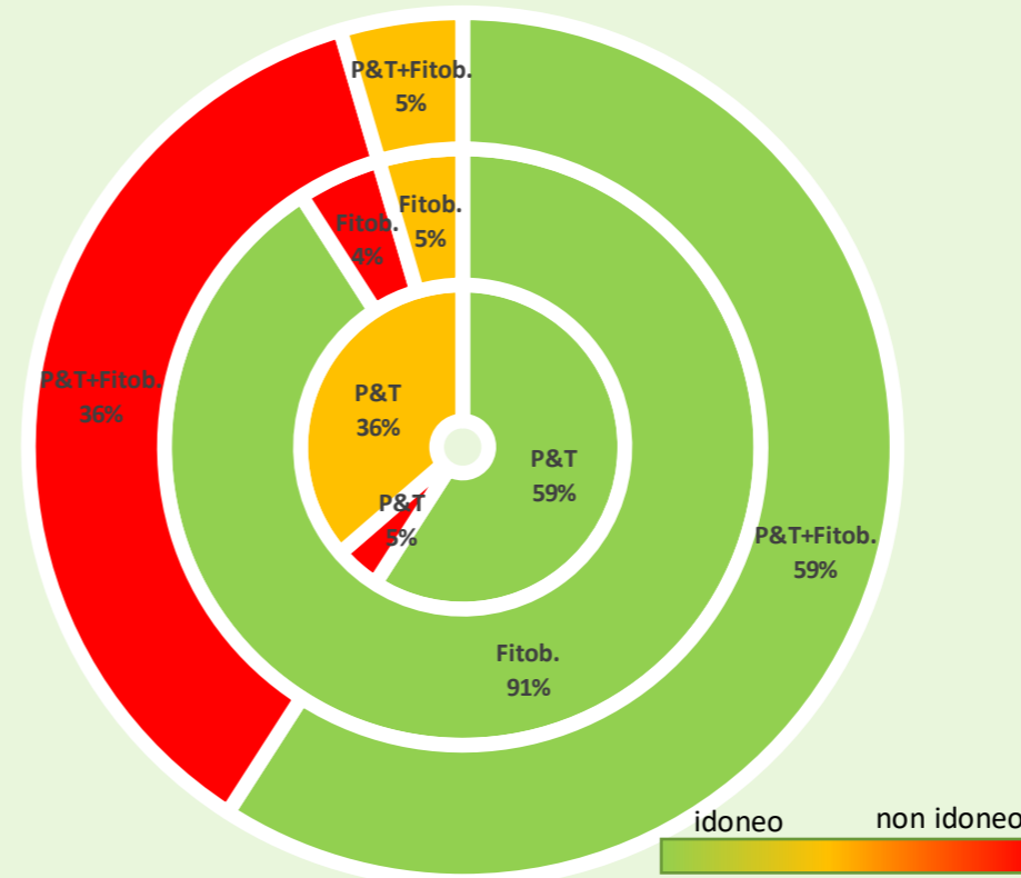
Diagramma ad anelli per la selezione della tecnologia zona saturata
