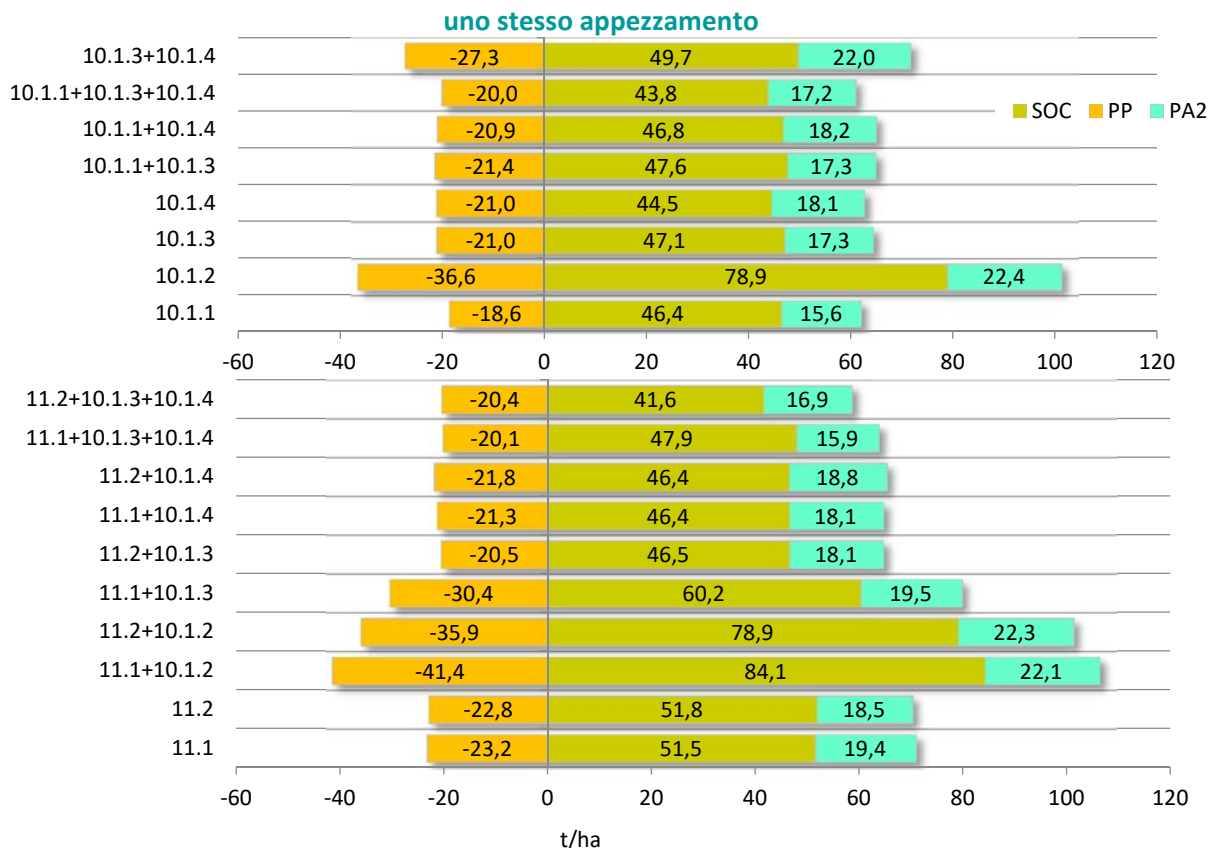
Fig. 53. Stock iniziale di C organico medio per ettaro, potenziale di accumulo (PA2) e di perdita (PP) dei suoli delle superfici ammesse a finanziamento distinte per insieme di interventi cumulati su uno stesso appezzamento
