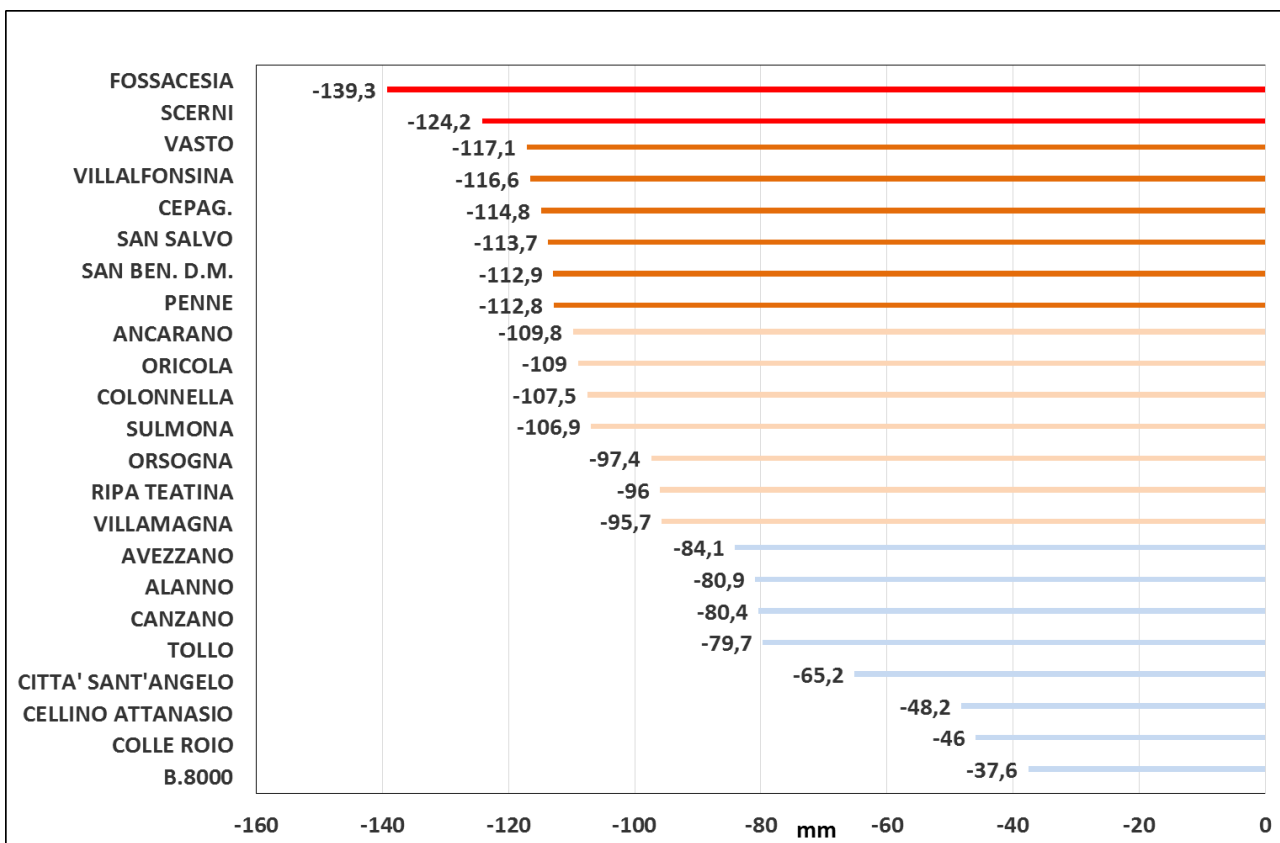
Fig. 15 Bilancio idrico climatico del mese di Agosto 2020
