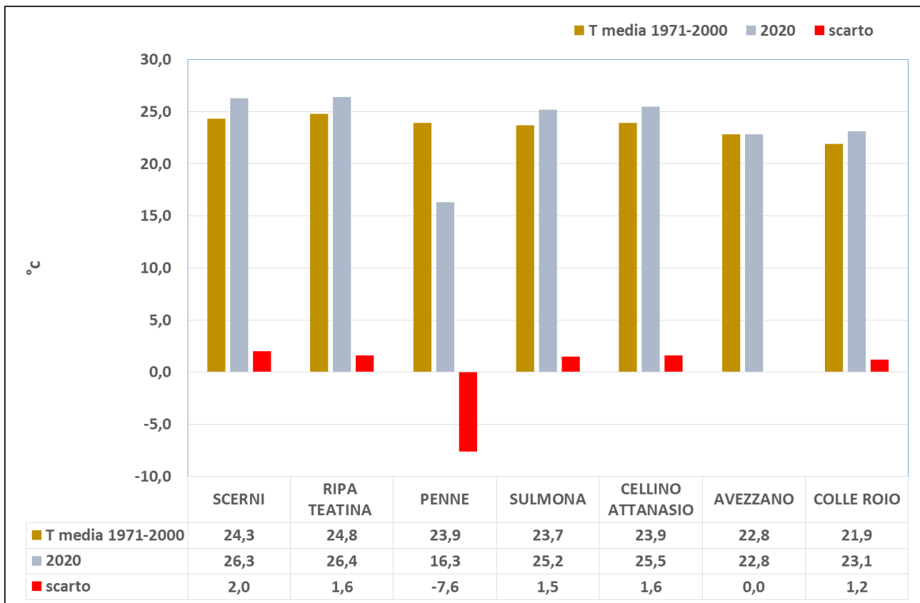
Fig. 3 Confronto per alcune località tra le temperature medie registrate nel mese di Agosto 2020 con quelle storiche (1971-2000). Per le località di Ripa Teatina, Cellino Attanasio e Colle Roio sono stati utilizzati per il confronto i dati termici rispettivamente di Chieti, Teramo e L'Aquila.
