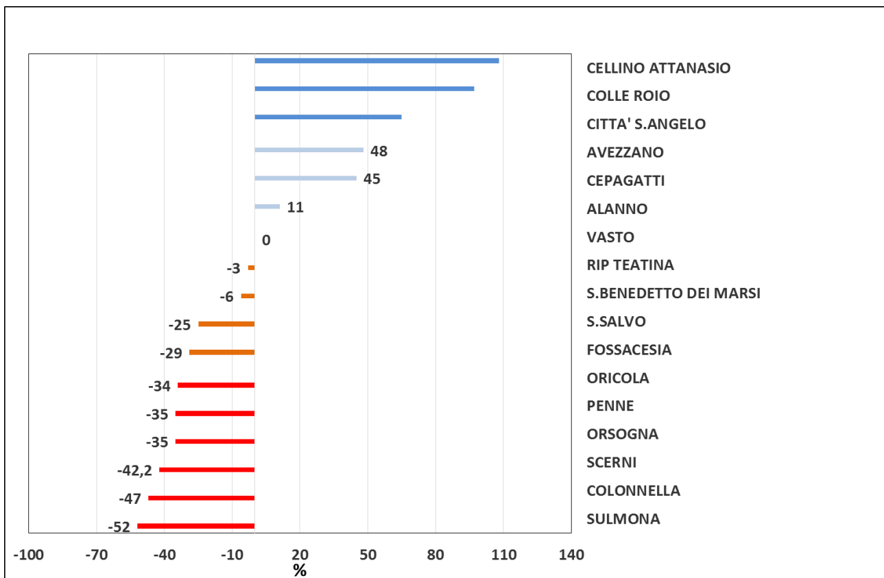
Fig. 12 Scarti in percentuale delle precipitazioni cumulate del mese di Agosto 2020 rispetto al dato storico (media 1971-2000).
