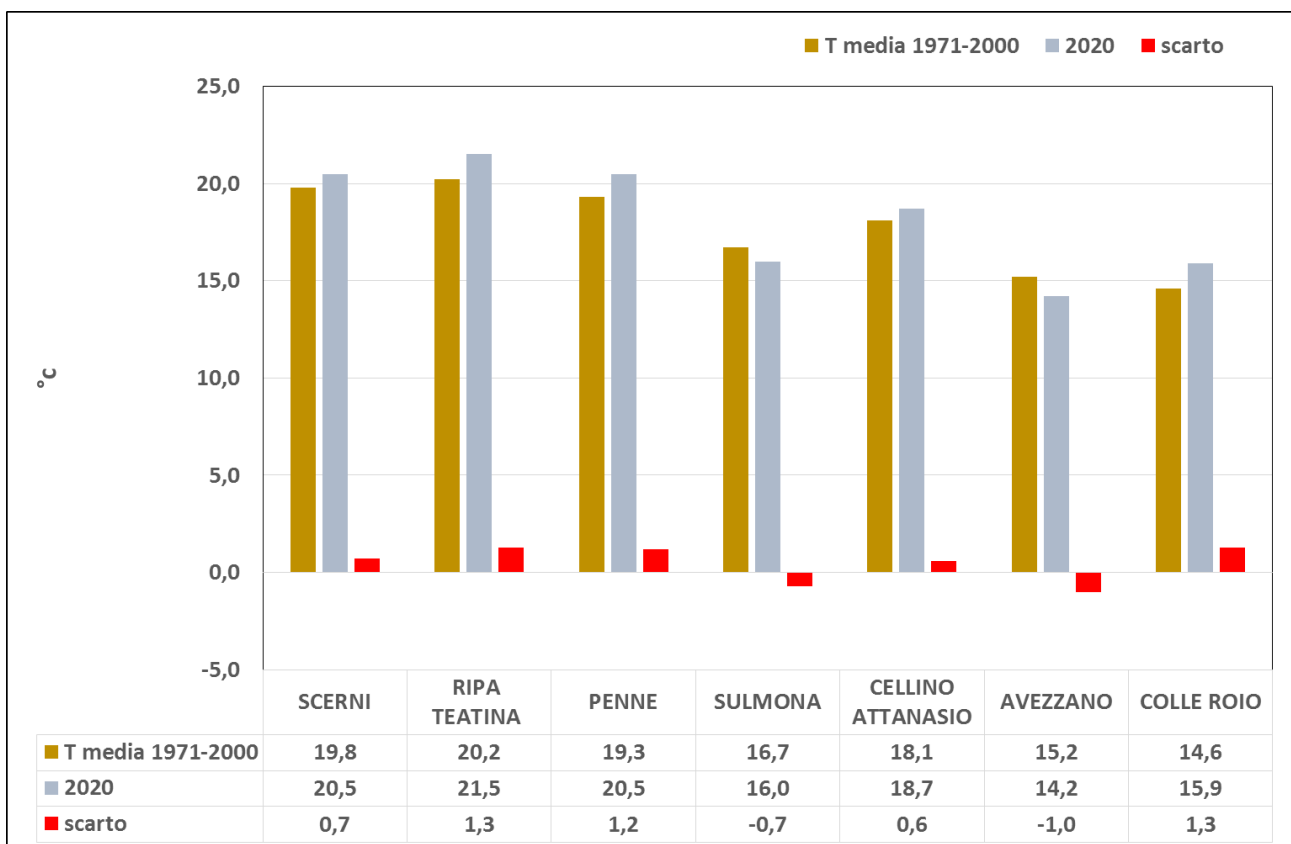
Fig. 7 Confronto per alcune località tra le medie delle temperature minime registrate nel mese di Agosto 2020 con quelle storiche (1971-2000). Per le località di Ripa Teatina, Colle Roio e Cellino Attanasio sono stati utilizzati per il confronto i dati termici rispettivamente di Chieti e L'Aquila e Teramo
