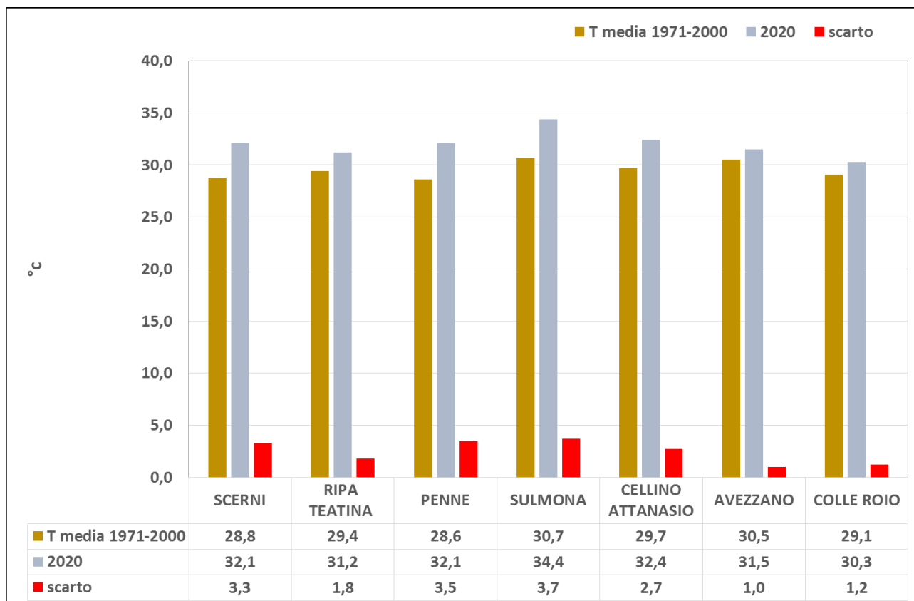
Fig. 5 Confronto per alcune località della regione Abruzzo tra le medie delle temperature massime registrate nel mese di Agosto 2020 con quelle storiche (1971-2000). Per le località di Ripa Teatina, Cellino Attanasio e Colle Roio e sono stati utilizzati per il confronto i dati termici rispettivamente di Chieti, Teramo e L’Aquila.
