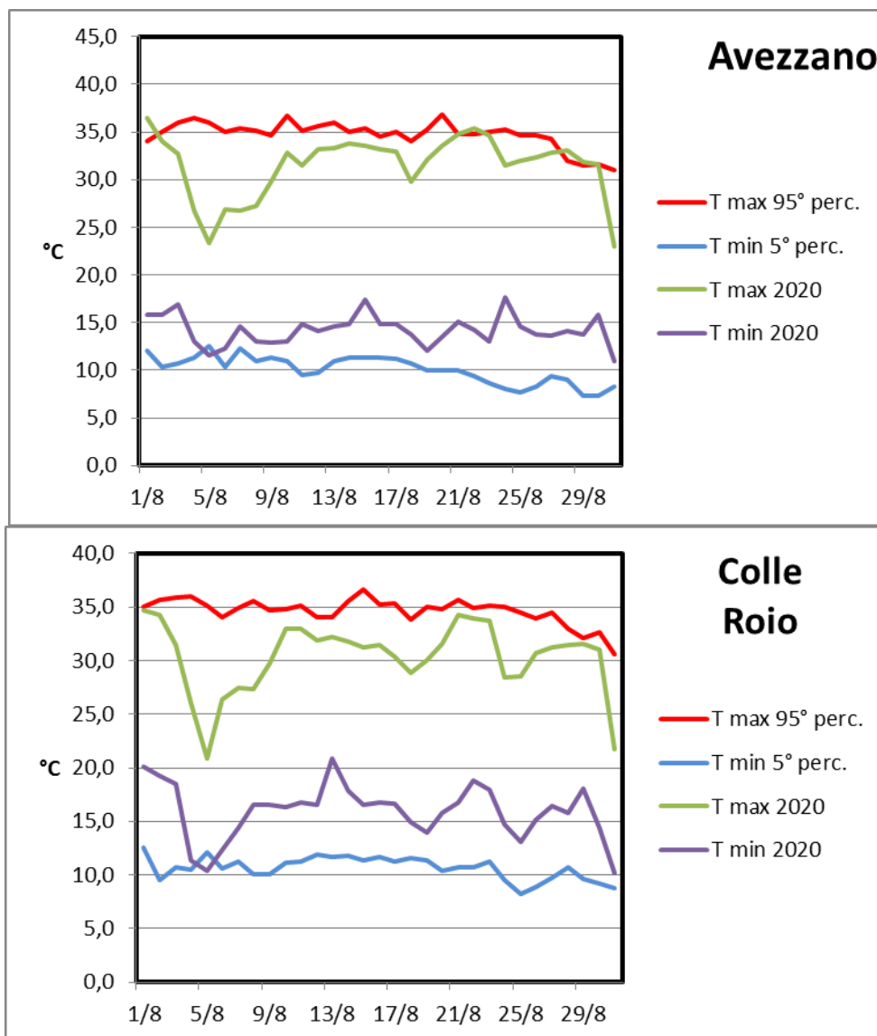
Fig.10 Confronto tra le temperature registrate nel mese di Agosto con il 5° percentile delle temperature minime e il 95° percentile delle temperature massime (serie storica 1971-2000). Per le località di Ripa Teatina, Colle Roio, Cellino Attanasio e Ancarano sono stati utilizzati per il confronto i dati termici rispettivamente di Chieti, L'Aquila, Teramo e Nereto
