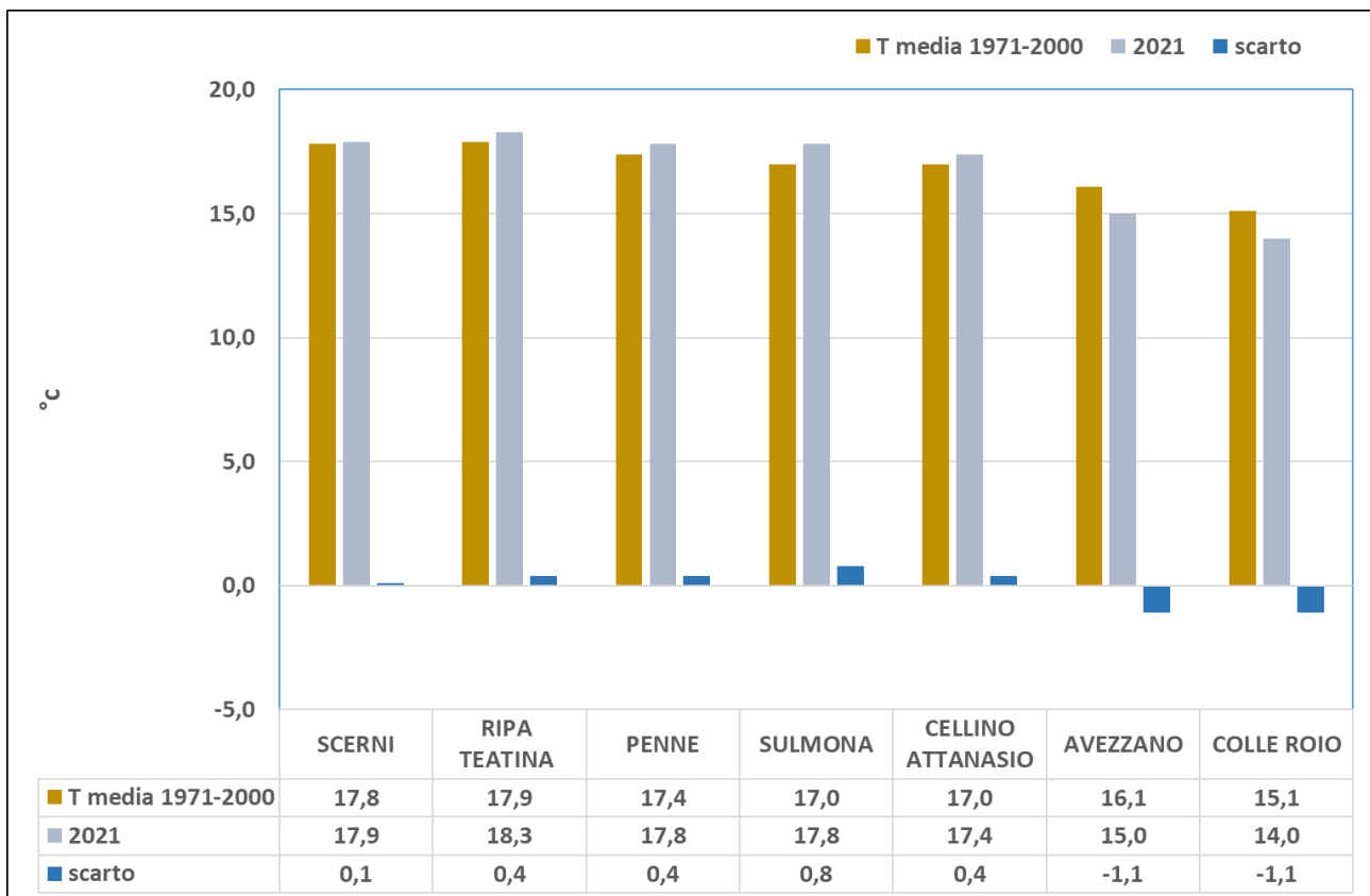
Fig. 3 Confronto per alcune località tra le temperature medie registrate nel mese di maggio 2021 con quelle storiche (1971-2000). Per le località di Ripa Teatina, Cellino Attanasio e Colle Roio sono stati utilizzati per il confronto i dati termici rispettivamente di Chieti, Teramo e L'Aquila.
