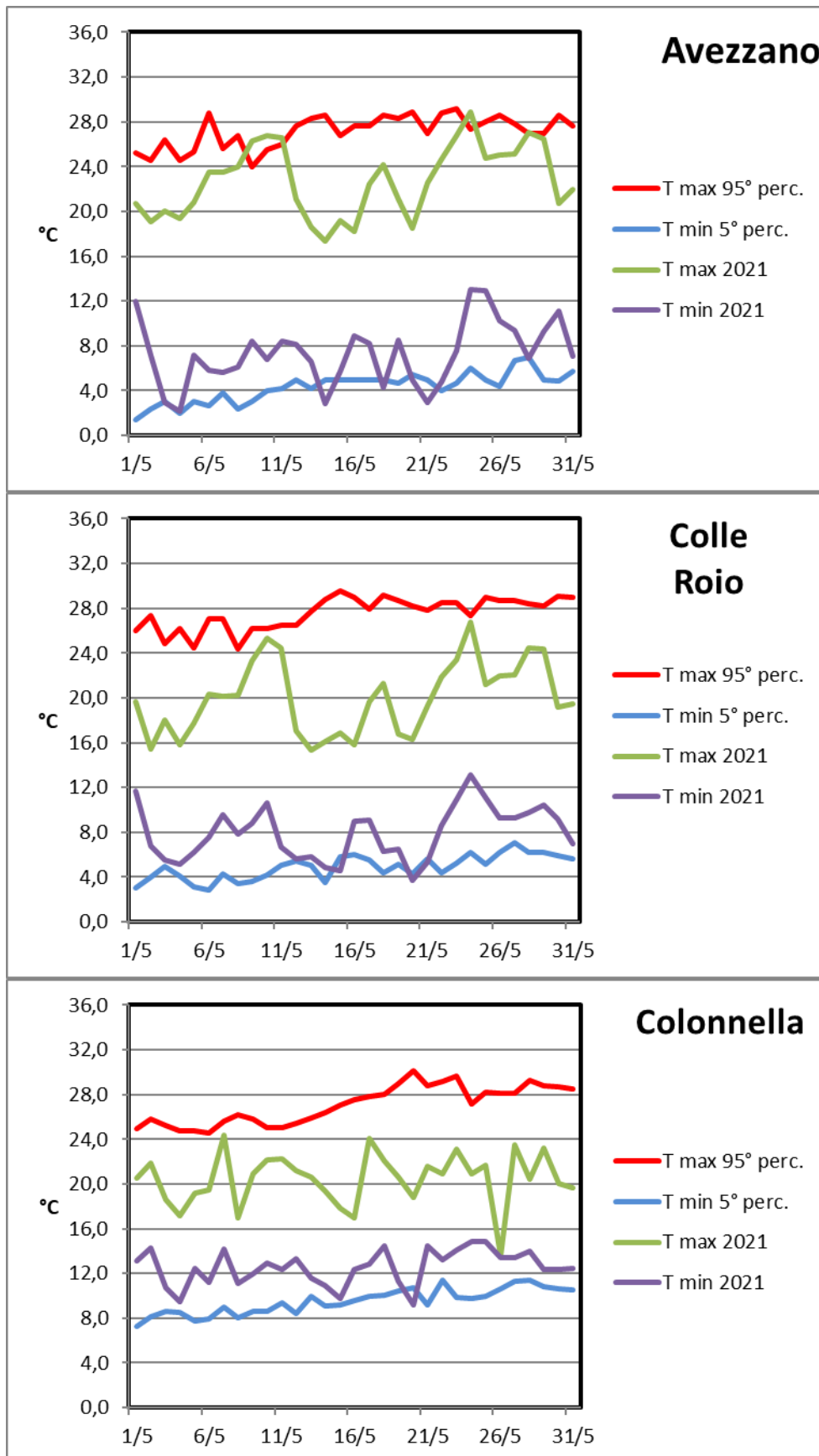
Fig.10 Confronto tra le temperature registrate nel mese di maggio con il 5° percentile delle temperature minime e il 95° percentile delle temperature massime (serie storica 1971-2000). Per le località di Ripa Teatina, Colle Roio, Cellino Attanasio e Ancarano sono stati utilizzati per il confronto i dati termici rispettivamente di Chieti, L'Aquila, Teramo e Nereto
