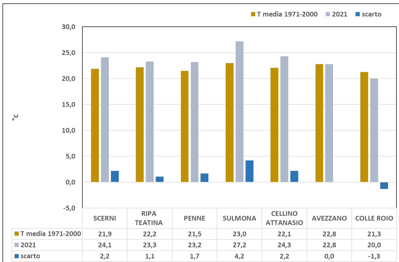
Fig. 5 Confronto per alcune località della regione Abruzzo tra le medie delle temperature massime registrate nel mese di maggio 2021 con quelle storiche (1971-2000). Per le località di Ripa Teatina, Cellino Attanasio e Colle Roio e sono stati utilizzati per il confronto i dati termici rispettivamente di Chieti, Teramo e L’Aquila.
