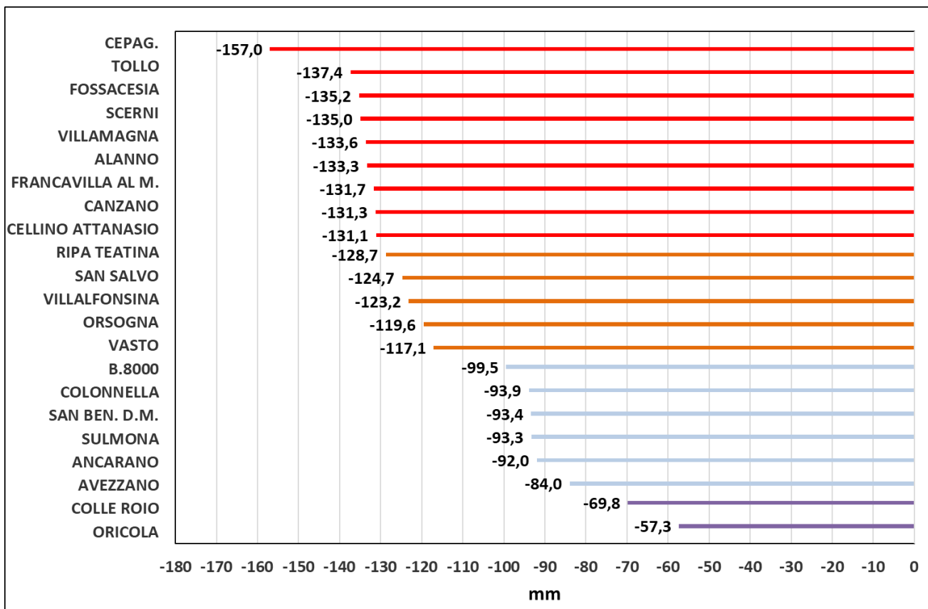
Fig. 15 Bilancio idrico climatico del mese di maggio 2021
