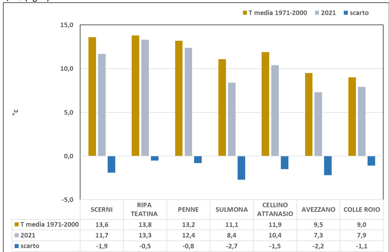
Fig. 7 Confronto per alcune località tra le medie delle temperature minime registrate nel mese di maggio 2021 con quelle storiche (1971-2000). Per le località di Ripa Teatina, Colle Roio e Cellino Attanasio sono stati utilizzati per il confronto i dati termici rispettivamente di Chieti e L'Aquila e Teramo
