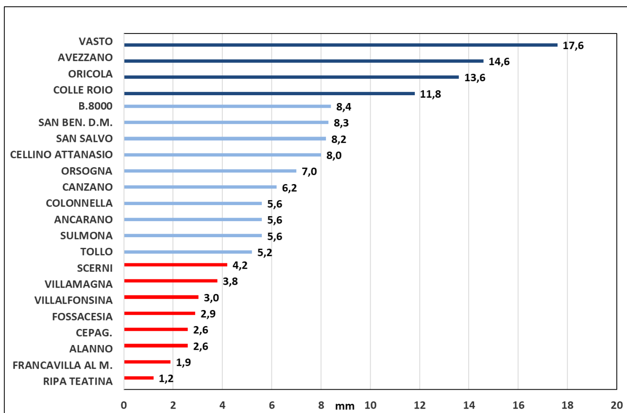
Fig. 13 Precipitazioni massime giornaliere
