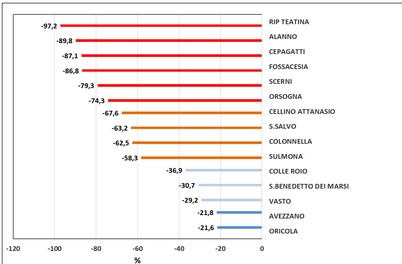
Fig. 12 Scarti in percentuale delle precipitazioni cumulate del mese di maggio 2021 rispetto al dato storico (media 1971-2000).
