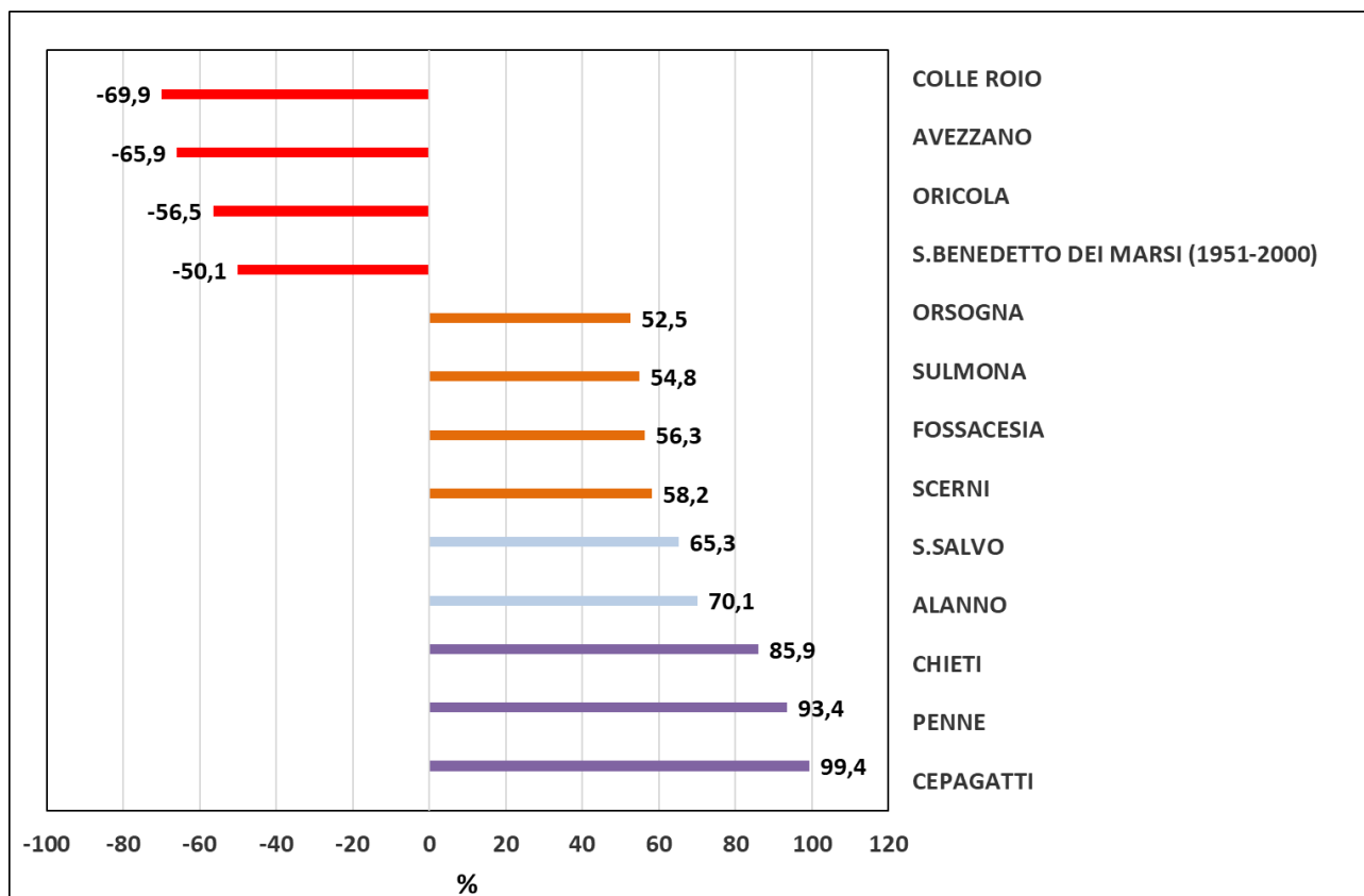
Fig. 12 Scarti in percentuale delle precipitazioni cumulate del mese di febbraio 2022 rispetto al dato storico (media 1971-2000). Le precipitazioni di Colle Roio e Fossacesia sono state confrontate con quelle dell'Aquila e Lanciano
