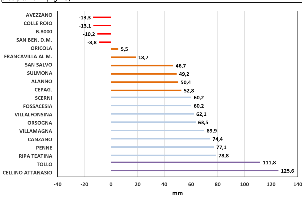
Fig. 15 Bilancio idrico climatico del mese di febbraio 2022
