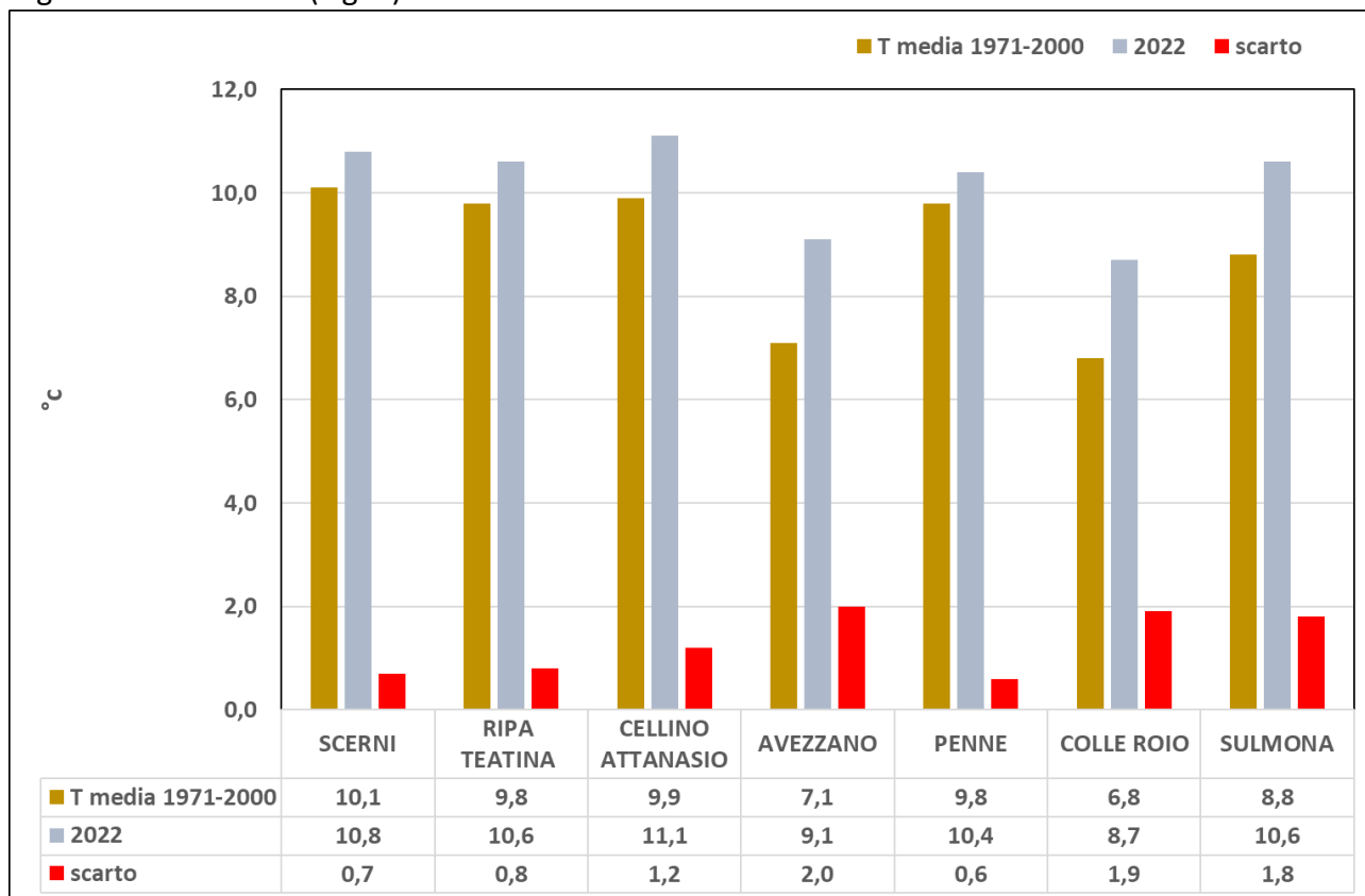
Fig. 5 Confronto per alcune località della regione Abruzzo tra le medie delle temperature massime registrate nel mese di febbraio 2022 con quelle storiche (1971-2000). Per le località di Ripa Teatina, Cellino Attanasio e Colle Roio e sono stati utilizzati per il confronto i dati termici rispettivamente di Chieti, Teramo e L'Aquila.
