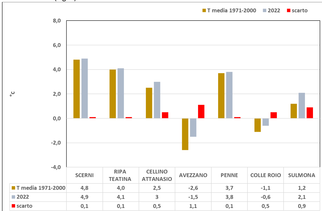
Fig. 7 Confronto per alcune località tra le medie delle temperature minime registrate nel mese di febbraio 2022 con quelle storiche (1971-2000). Per le località di Ripa Teatina, Colle Roio e Cellino Attanasio sono stati utilizzati per il confronto i dati termici rispettivamente di Chieti e L'Aquila e Teramo
