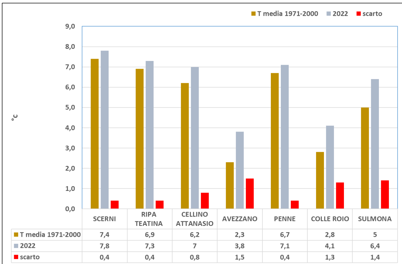
Fig. 3 Confronto per alcune località tra le temperature medie registrate nel mese di febbraio 2022 con quelle storiche (1971-2000). Per le località di Ripa Teatina, Cellino Attanasio e Colle Roio sono stati utilizzati per il confronto i dati termici rispettivamente di Chieti, Teramo e L'Aquila.
