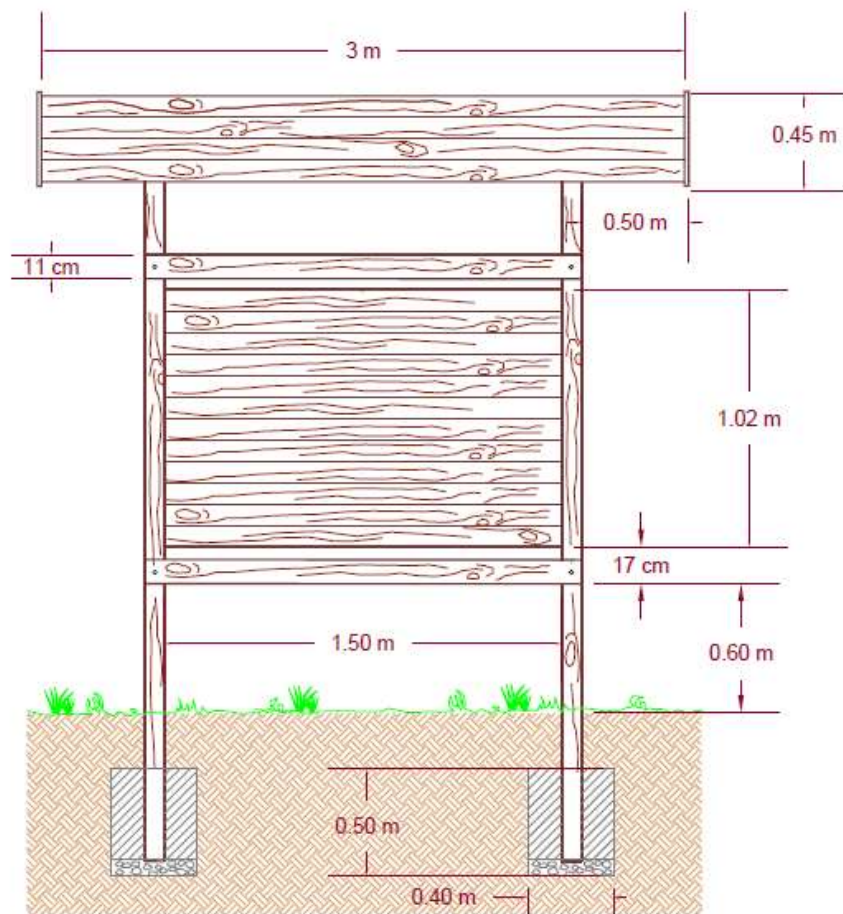
Prospetto frontale
