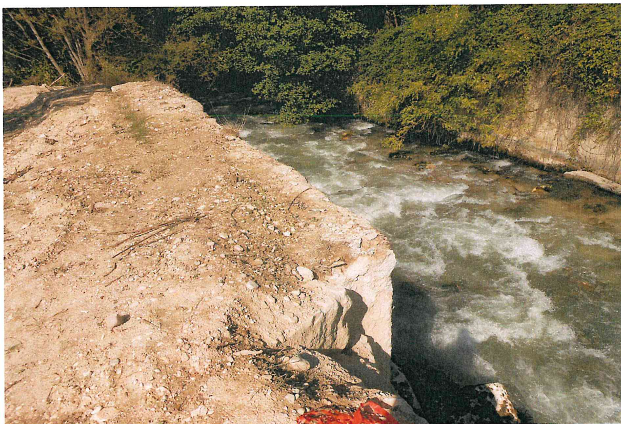
foto 2 vista del muro d'argine in sx idraulica danneggiato
