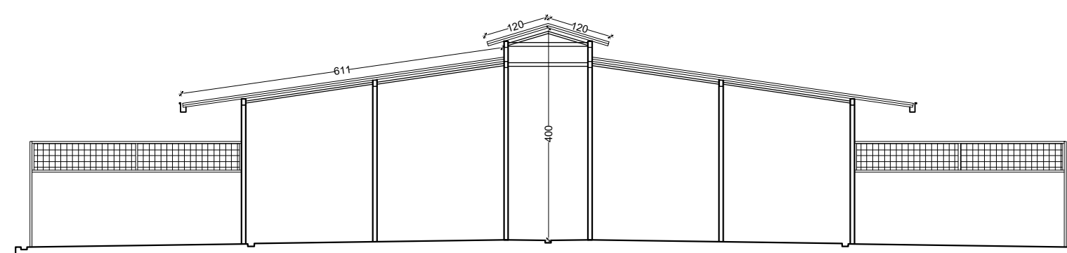
Sezione tipo Box Cani - Scala 1:100
