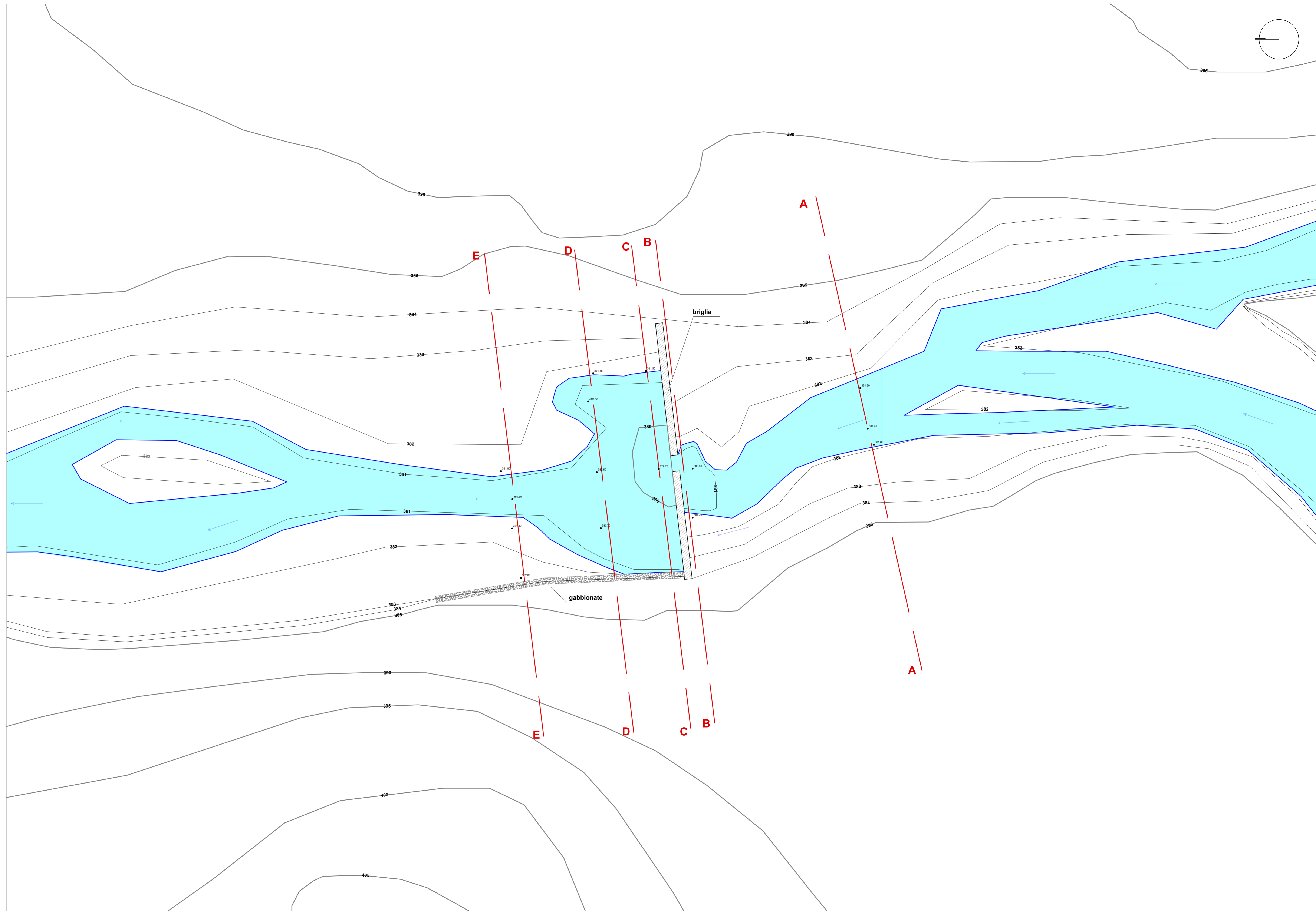
Rilievo piano-altimetrico (Scala 1:250)
