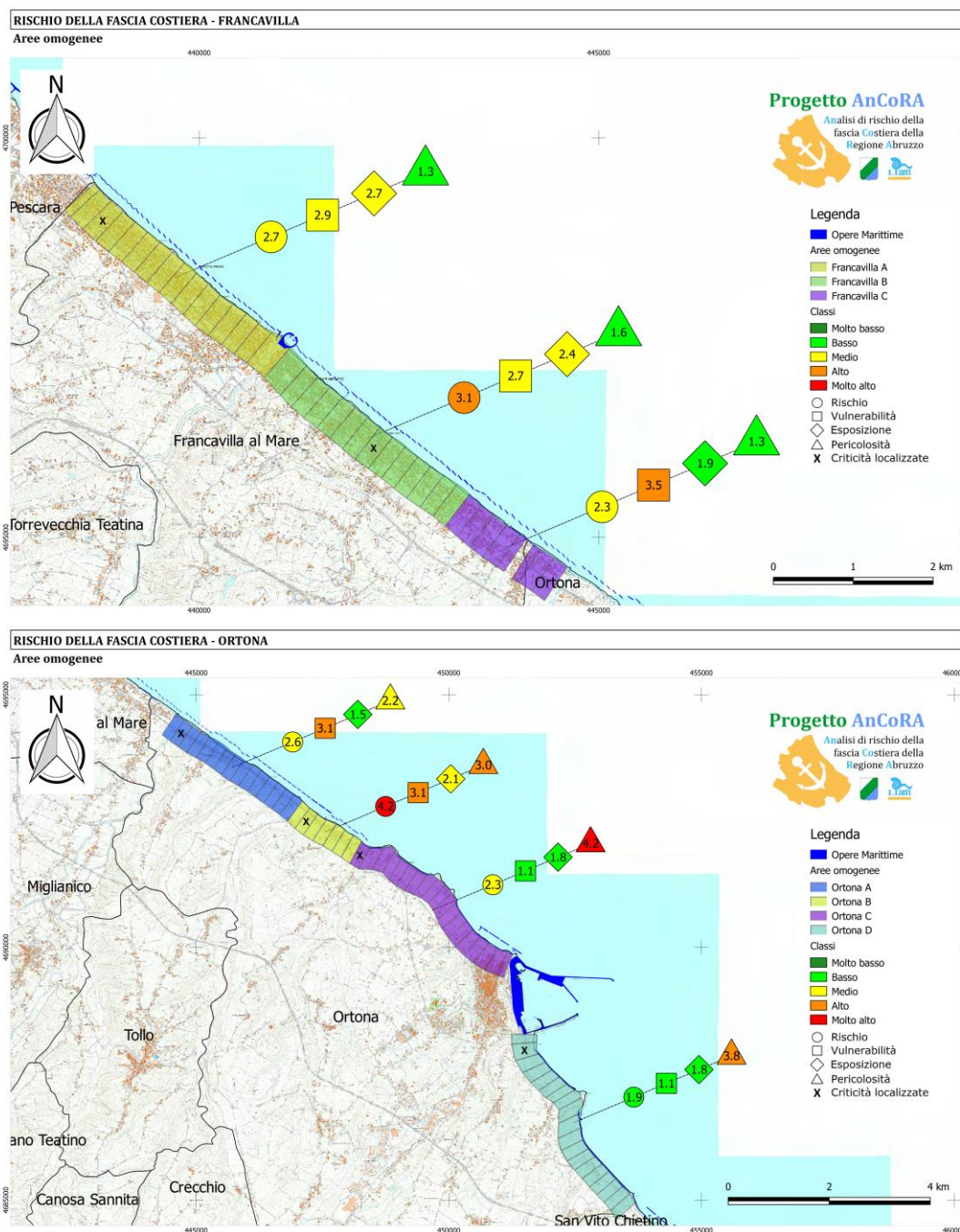
Figura 7-1: Sintesi dei risultati dell'analisi di rischio. Area compresa tra la Darsena di Francavilla e il centro abitato di Ortona (mappa in alto) e tra il centro abitato di Francavilla e Torre Mucchia (mappa in basso). Valutazione della vulnerabilità (numero nel contorno quadrato), dell'esposizione (numero nel contorno romboidale), della pericolosità (numero nel contorno triangolare) e del rischio (numero nel contorno tondo).
