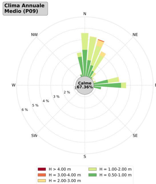
Figura 4-18: Propagazione del moto ondoso sotto costa. Anno climatico medio. Rappresentazione polare della frequenza di apparizione (lunghezza delle barre) degli eventi di moto ondoso sotto costa in funzione dell'altezza d'onda significativa (colori) e della direzione di provenienza. Le calme sono costituite dagli eventi con altezza d'onda significativa strettamente inferiore al valore 0.50 m. (3/3)
