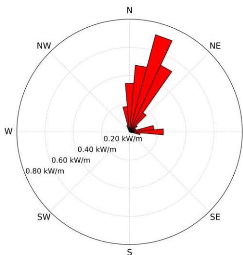
Flusso Energetico Medio a costa (P05)
