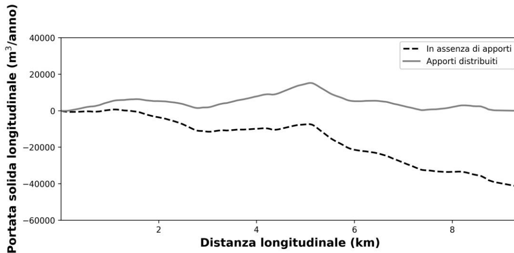
Figura 6-6: Analisi della tendenza evolutiva recente del litorale. Stima morfologica della portata solida longitudinale in assenza di apporto (linea tratteggiata), valutata nell'ipotesi di apporti distribuiti uniformemente su tutto il litorale (linea grigia). La distanza longitudinale è definita con verso positivo verso Sud-Est ed origine posta in corrispondenza del limite Nord dell'Unità Fisiografica. Per facilità di lettura, la Tabella 6-1 esplicita le ascisse di alcuni punti notevoli lungo il litorale.
