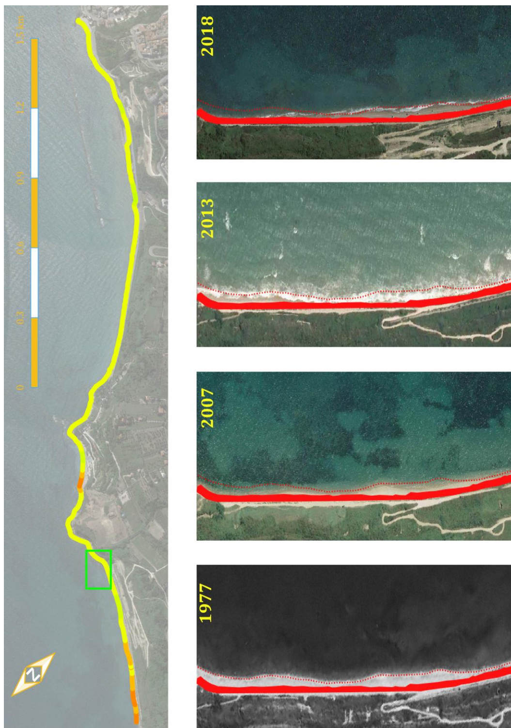
Figura 6-3: Analisi della tendenza evolutiva recente del litorale. Confronto delle ortofoto del 1997, 2007, 2013 e 2018 nell'area prossima alla Riserva Naturale Regionale "Ripari di Giobbe". La linea di riva riportata è quella relativa al 1997.
