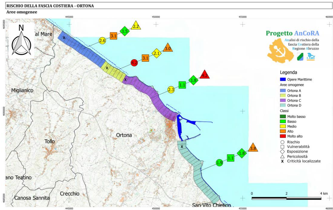
Figura 7-1: Sintesi dei risultati dell'analisi di rischio. Area compresa tra Torre Mucchia e il porto di Ortona (mappa in alto). Valutazione della vulnerabilità (numero nel contorno quadrato), dell'esposizione (numero nel contorno romboidale), della pericolosità (numero nel contorno triangolare) e del rischio (numero nel contorno tondo).
