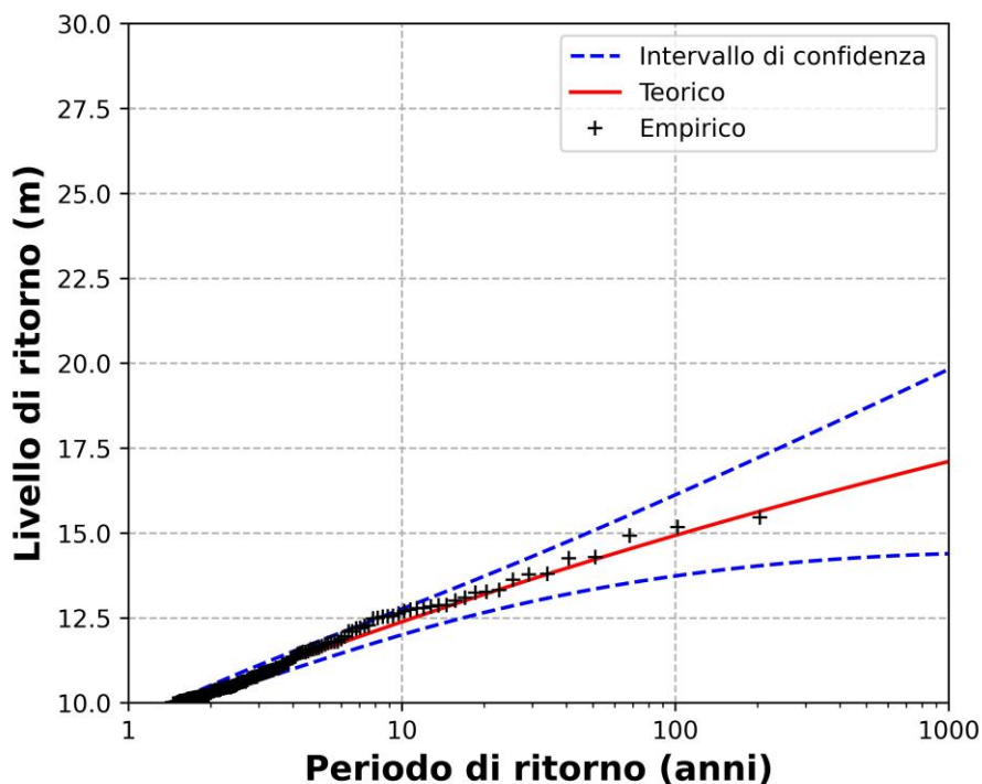
Figura 4-5: Risultati dell'analisi anemometrica. Analisi estrema. Settore di traversia secondario (Levante-Scirocco-Mezzogiorno, 70°N-200°N). Variazione del livello di ritorno (intensità del vento) in funzione del tempo di ritorno.
