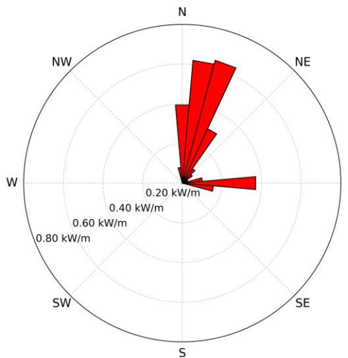
Flusso Energetico Medio a costa (P11)
