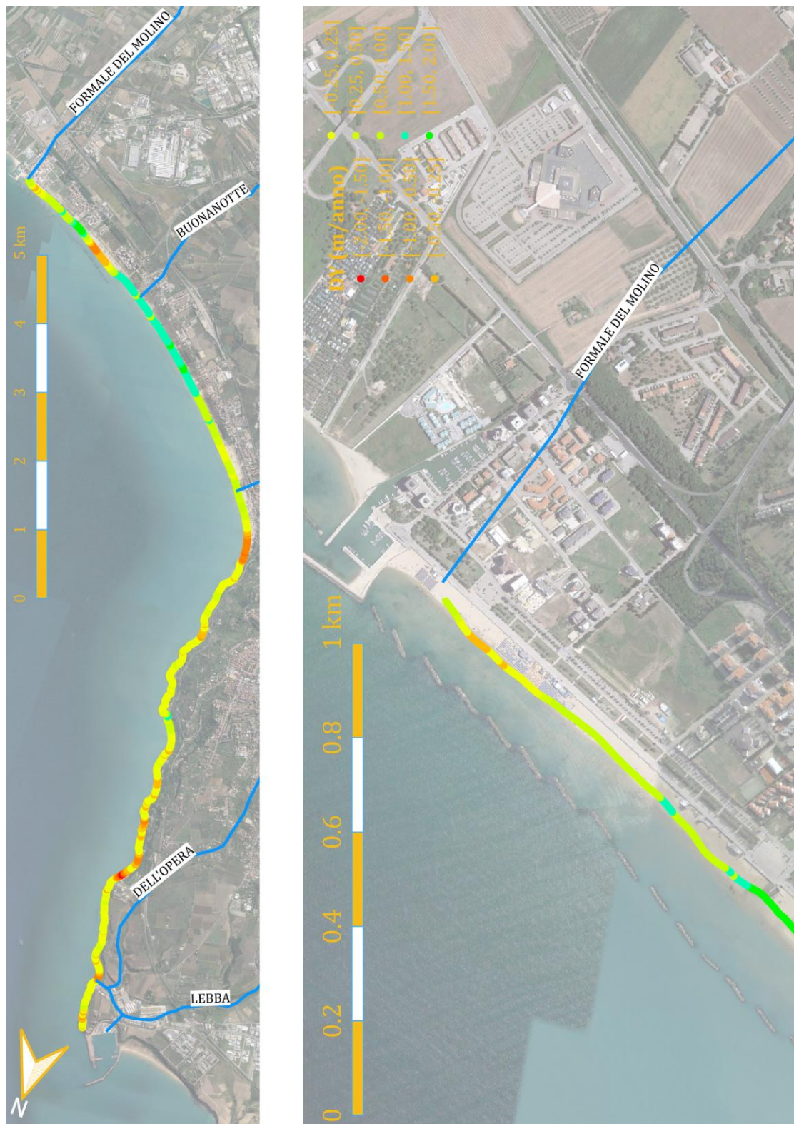
Figura 6-7: Analisi della tendenza evolutiva recente del litorale. Evoluzione della linea di riva nel periodo 1997-2018. Dettaglio tra il centro di San Salvo Marina e la foce del Trigno.
