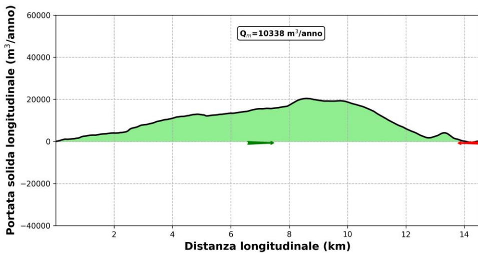
Figura 6-11: Analisi della tendenza evolutiva recente del litorale. Stima morfologica della portata solida longitudinale. La distanza longitudinale è definita con verso positivo verso Sud-Est ed origine posta in corrispondenza del limite Nord dell'Unità Fisiografica. Per facilità di lettura, la Tabella 6-1 esplicita le ascisse di alcuni punti notevoli lungo il litorale.
