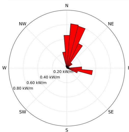
Flusso Energetico Medio a costa (P08)
