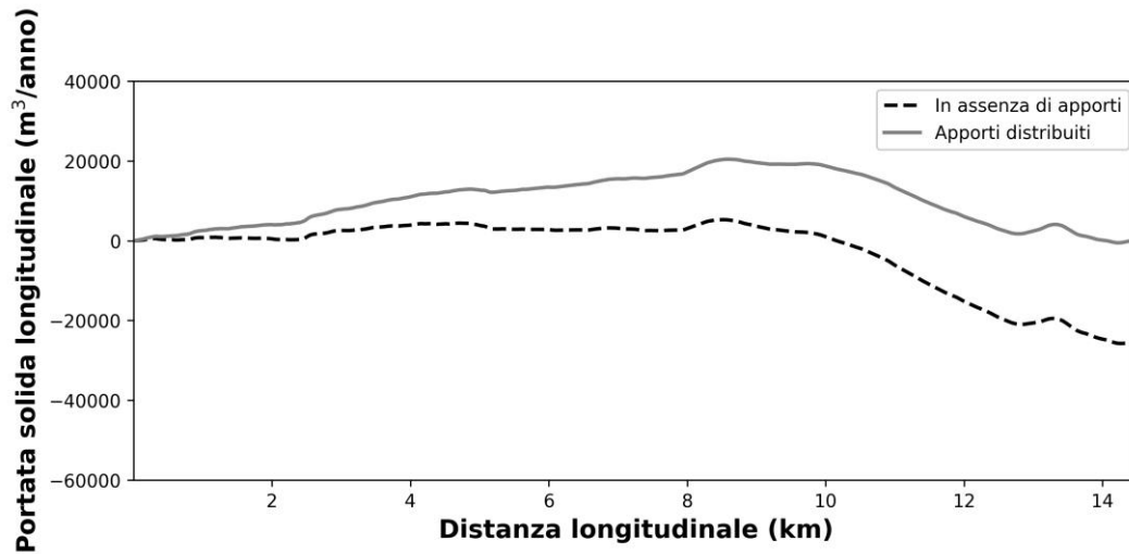
Figura 6-10: Analisi della tendenza evolutiva recente del litorale. Stima morfologica della portata solida longitudinale in assenza di apporto (linea tratteggiata), valutata nell'ipotesi di apporti distribuiti uniformemente su tutto il litorale (linea grigia) e valutata nell'ipotesi di apporti concentrati in corrispondenza delle foci fluviali. La distanza longitudinale è definita con verso positivo verso Sud-Est ed origine posta in corrispondenza del limite Nord dell'Unità Fisiografica. Per facilità di lettura, la Tabella 6-1 esplicita le ascisse di alcuni punti notevoli lungo il litorale.
