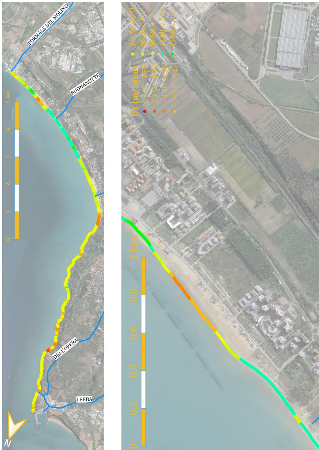
Figura 6-6: Analisi della tendenza evolutiva recente del litorale. Evoluzione della linea di riva nel periodo 1997-2018. Dettaglio tra la Foce del fosso Buonanotte e il centro di San Salvo Marina.
