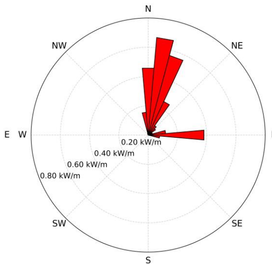
Flusso Energetico Medio a costa (P12)
