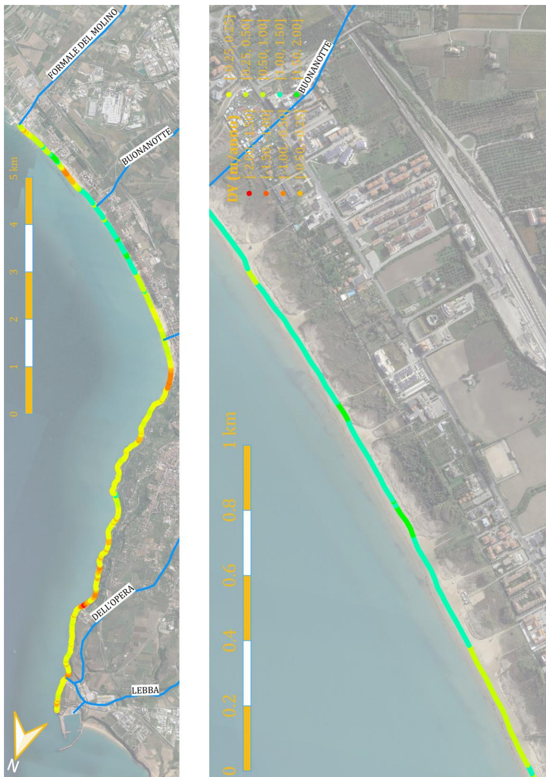
Figura 6-5: Analisi della tendenza evolutiva recente del litorale. Evoluzione della linea di riva nel periodo 1997-2018. Dettaglio tra il centro di Vasto Marina e la foce del fosso Buonanotte.
