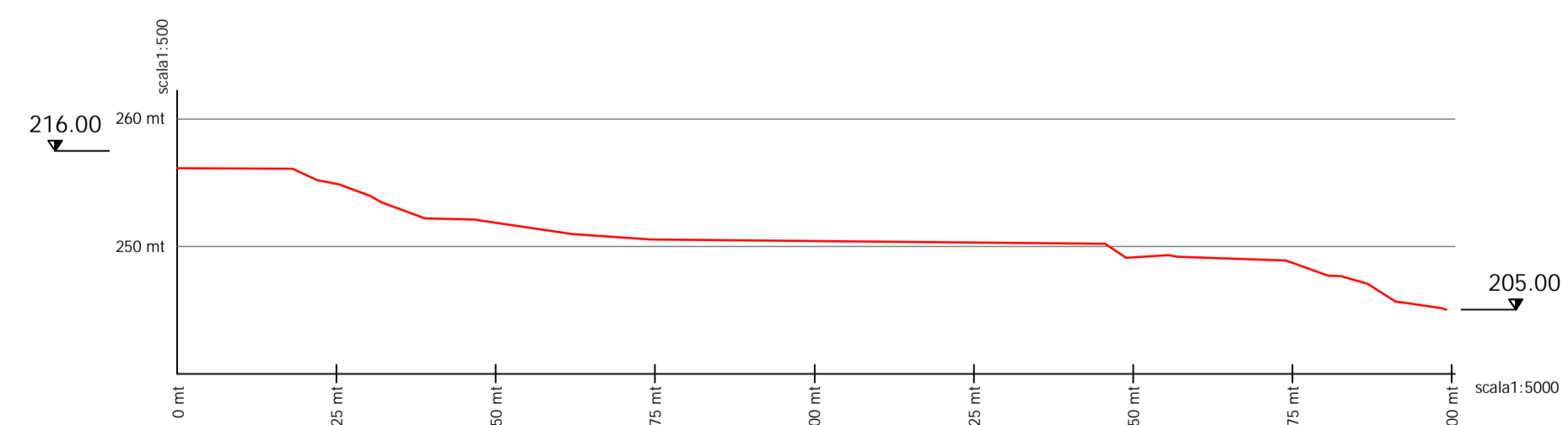
PROFILO nodo 305 - 302 Salto mt. 11.00 Lunghezza mt. 995.76
