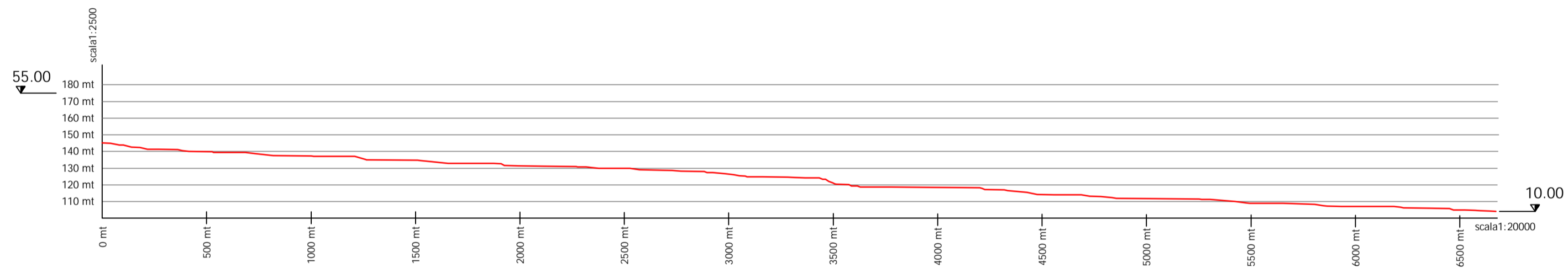
PROFILO nodo 257 - 231 Salto mt. 45.00 Lunghezza mt. 7096.82
