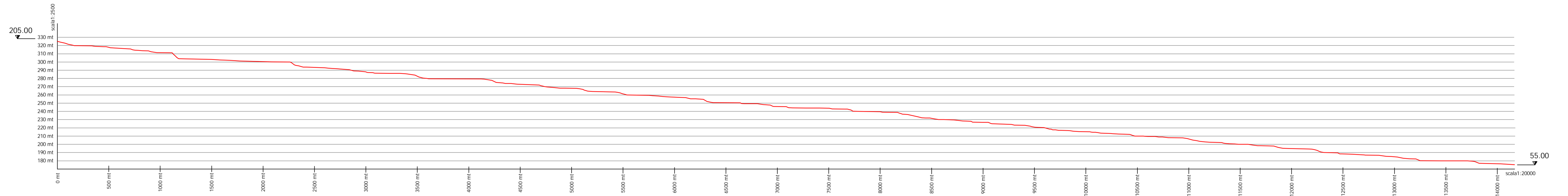
PROFILO nodo 302 - 257 Salto mt. 150.00 Lunghezza mt. 14166.94
