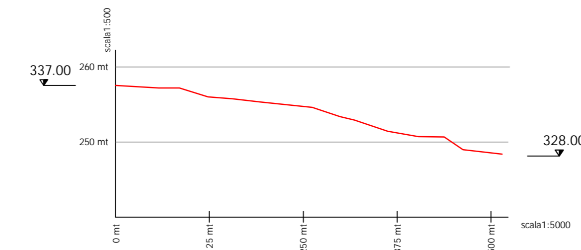
PROFILO nodo 449 - 445 Salto mt. 9.00 Lunghezza mt. 514.90
