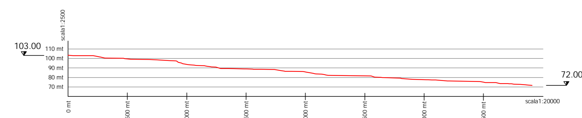
PROFILO nodo 410 - 405 Salto mt. 31.00 Lunghezza mt. 3910.20
