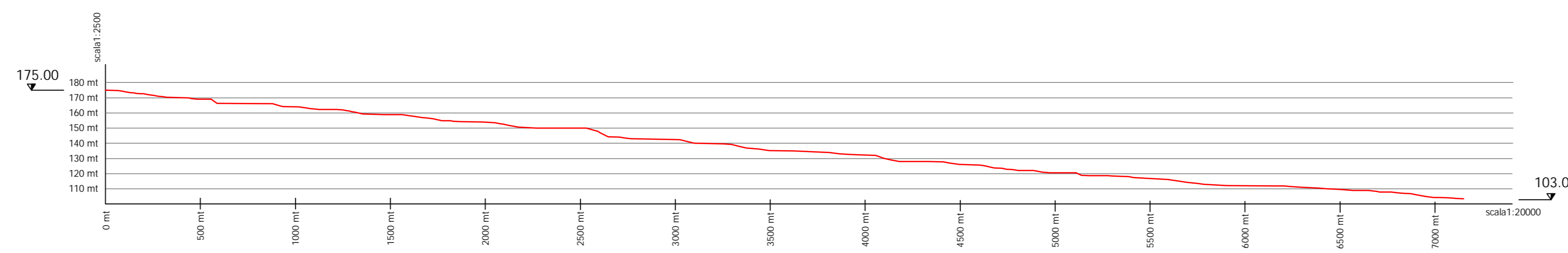
PROFILO nodo 428 - 410 Salto mt. 72.00 Lunghezza mt. 7151.40
