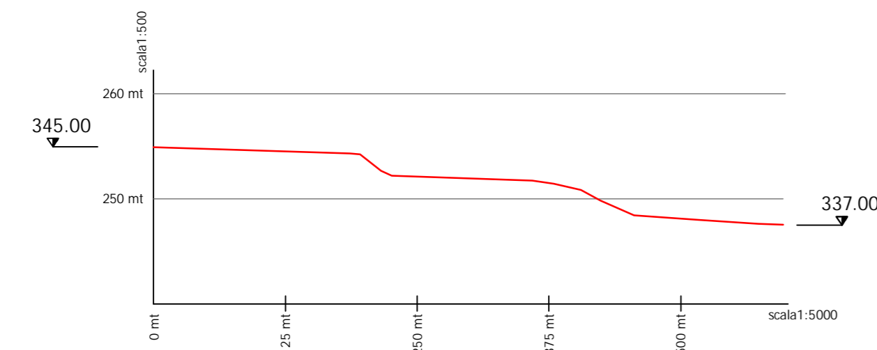
PROFILO nodo 451 - 449 Salto mt. 8.00 Lunghezza mt. 596.99
