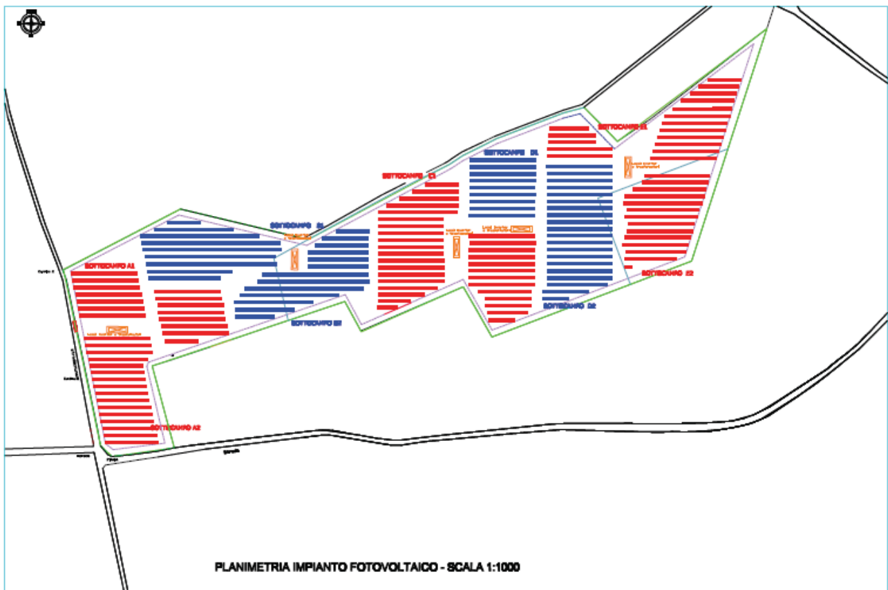
Figura 3: layout di impianto ove risulta visibile la viabilità perimetrale delle varie sezioni
